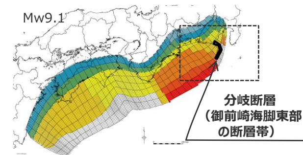
検討波源モデルB-2 (プレート境界面浅部・御前崎海脚東部の断層帯) の波源モデル
