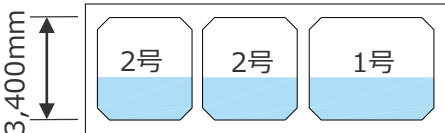
1,2号放水路標準断面図
