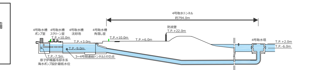
4号取水塔～4号取水トンネル～4号取水槽縦断面図
