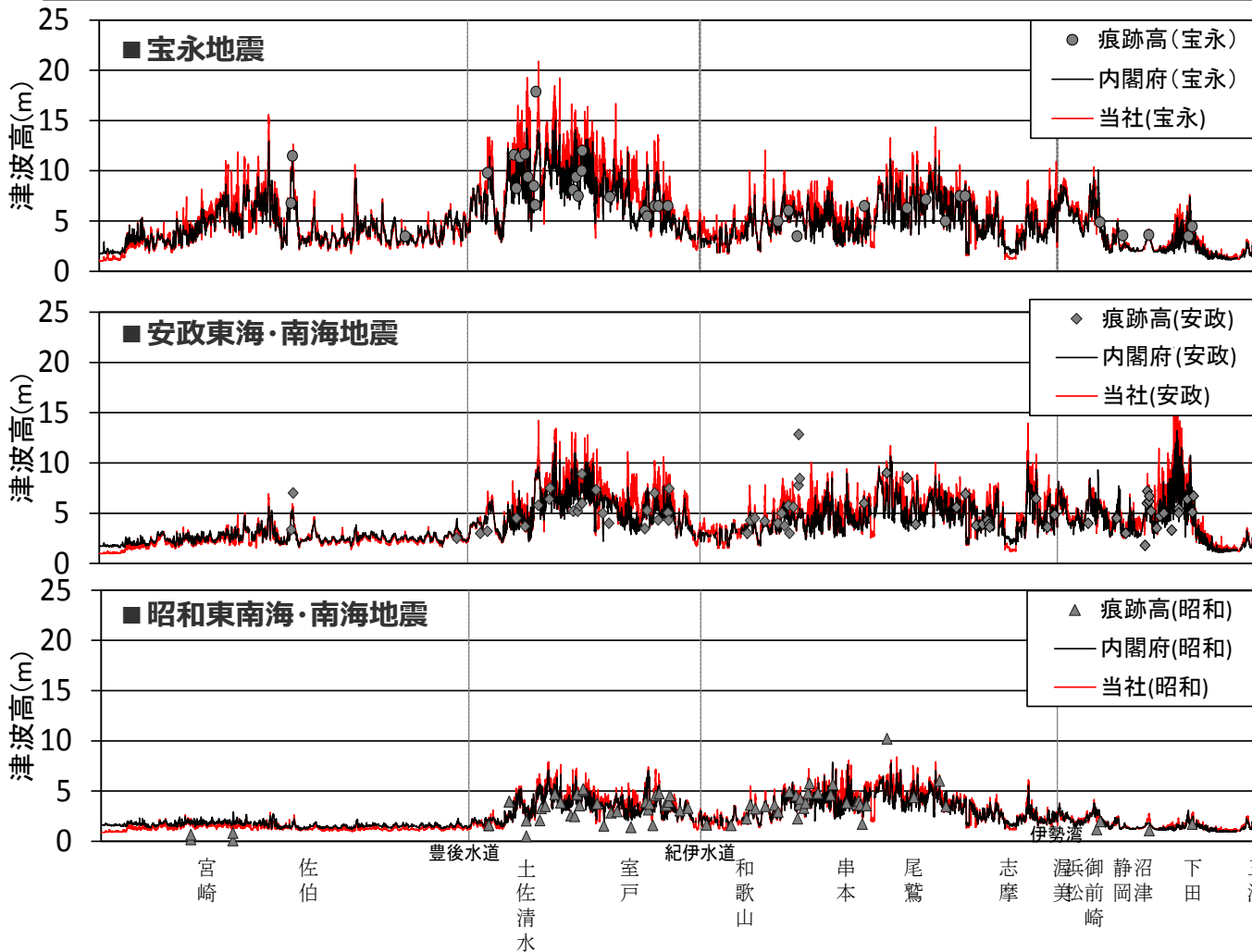
既往津波の再現性の確認 (津波痕跡高および内閣府(2015)の数値シミュレーション結果との比較)
