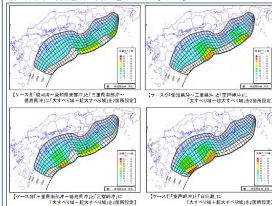
(内閣府(2012)を基に作成) 内閣府の最大クラスモデルの波源モデル (ケース①～⑪)
