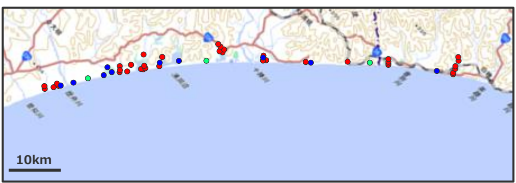
十勝周辺の調査地点 (内閣府(2020)を基に作成)
