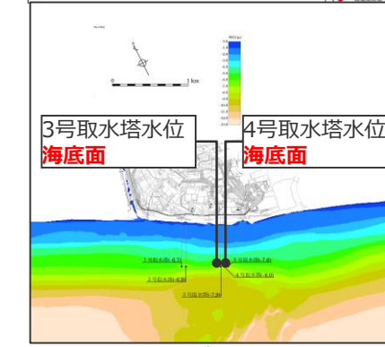
最大下降水位分布
