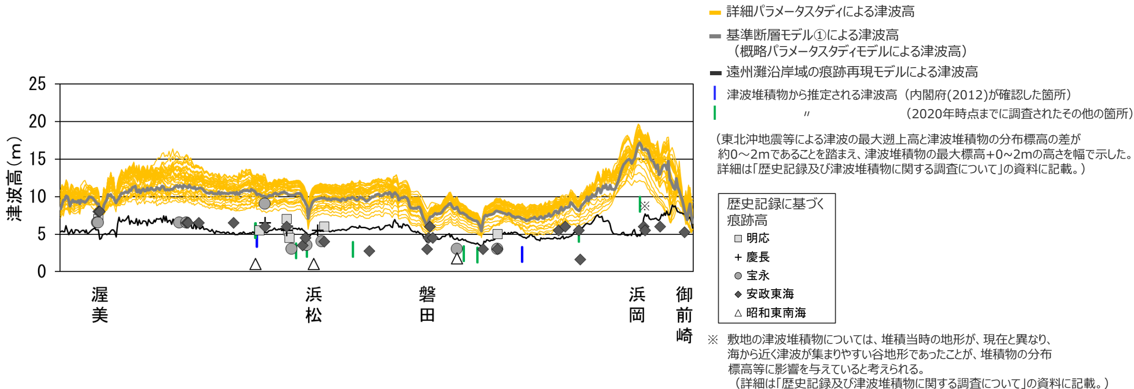
パラメータスタディによる海岸線の津波高と、歴史記録及び津波堆積物から推定される津波高との比較
