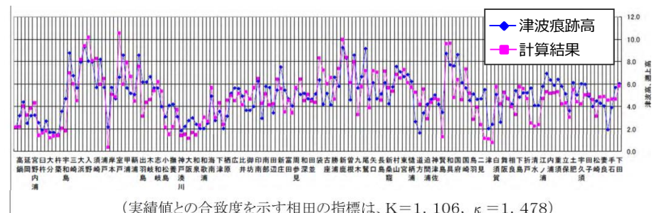
中央防災会議(2003)の津波痕跡再現モデルによる津波高と、 過去の5地震による津波痕跡高との比較
