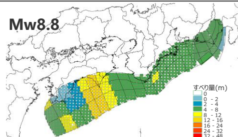
東海・東南海・南海地震モデル (中央防災会議(2003)に基づく)
