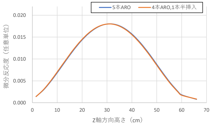
図 A-14 C45G0(4列)炉心のC2制御棒微分反応度曲線 (曲線の積分値が1となるように規格化) (青線：C2以外の5本の制御棒は全引抜き、 オレンジ線：C2と反対側のC1制御棒を半分まで挿入)
