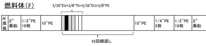
(a) 1/8"p41ETh燃料体
