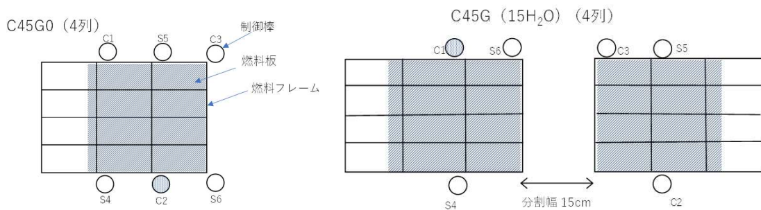
図 A-13 C45G0(4 列)炉心 C45G(15H 2 O) (4 列)炉心の配置図
