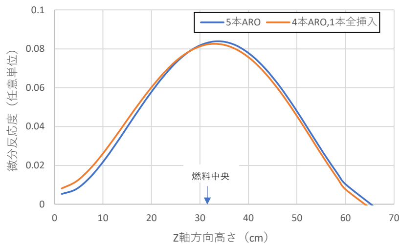
図 A-15 C45G(15H 2 O)(4列)炉心のC2制御棒微分反応度曲線 (曲線の積分値が1となるように規格化) (青線：C2以外の5本の制御棒は全引抜き、 オレンジ線：C2と反対側のS5制御棒を半分まで挿入)
