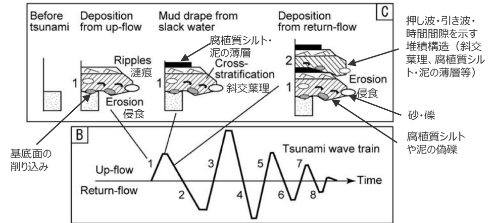
津波の押し波・引き波による津波堆積物の堆積プロセス
