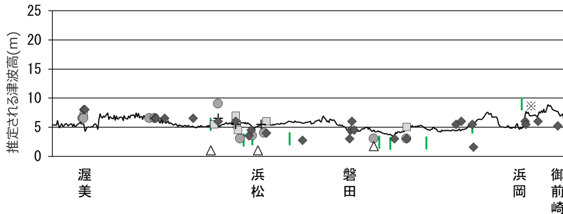
最大遡上高と津波堆積物の分布標高の関係を踏まえて推定される津波高
