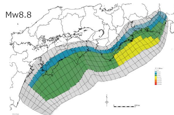
プレートの沈み込み速度を考慮したモデル (応力降下量 : 1.8MPa)
