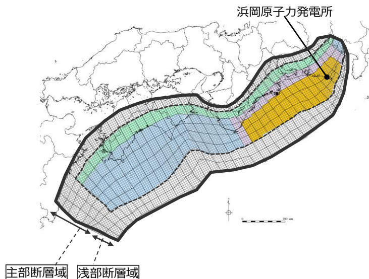
プレートの沈み込み速度を考慮しないモデル (応力降下量：1.5MPa)
