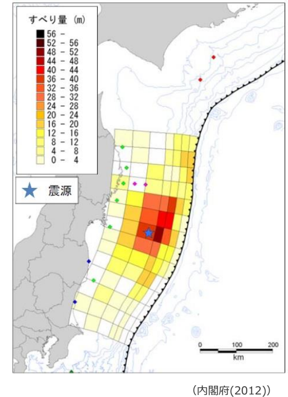
2011年東北沖地震のインバージョン結果に基づく波源モデル
