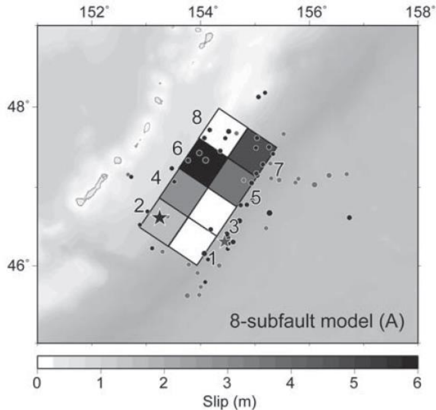
Fujii and Satake(2008a)による波源モデル
