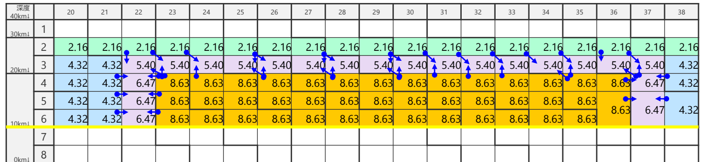
遷移領域のすべり量 D (m) の設定方法
