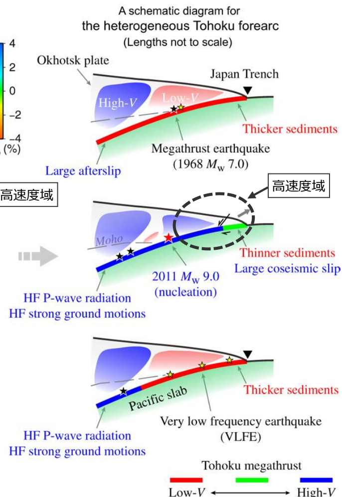
2011年東北沖地震の速度分布とそのイメージ (Liu and Zhao(2018)を基に作成)
