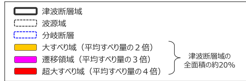
検討波源モデルB-2 (プレート境界面浅部・御前崎海脚東部の断層帯) の各小断層のすべり量分布 (m)
