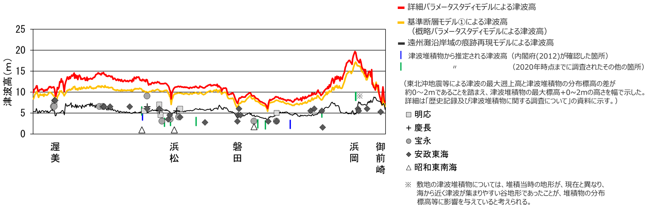
プレート間地震の波源モデルによる海岸線の津波高と、歴史記録及び津波堆積物から推定される津波高との比較
