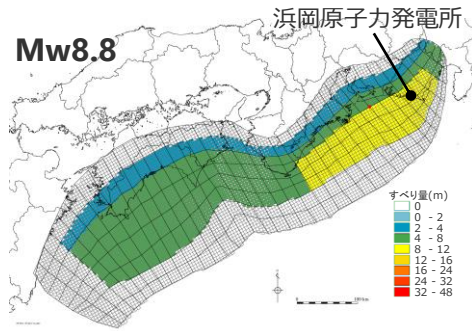
プレートの沈み込み速度を考慮しないモデル ( \Delta\sigma = 1.7\text{MPa} の例)
