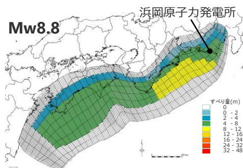
プレートの沈み込み速度を考慮したモデル ( \Delta\sigma = 1.7\text{MPa} の例)
