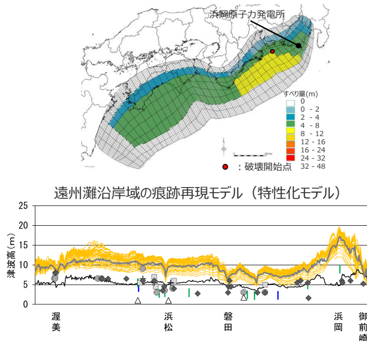
パラメータスタディによる海岸線の津波高と、歴史記録及び津波堆積物から推定される津波高との比較
