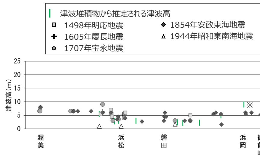
歴史記録及び津波堆積物から推定される遠州灘沿岸域の津波高
