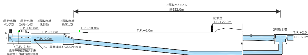
3号取水塔~3号取水トンネル~3号取水槽縦断面図
