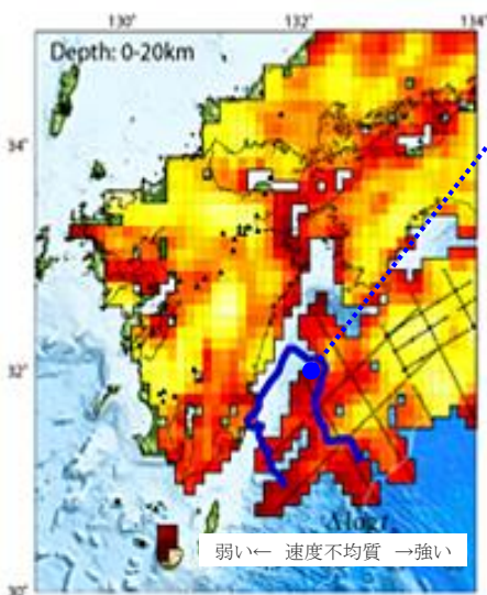
九州・パラオ海嶺での構造変化と南海トラフにおける地震に関する見解 (文部科学省・海洋研究開発機構 (2013)に加筆)
