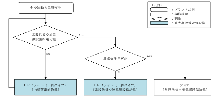
第 1.16-6 図 対応手段選択フローチャート
