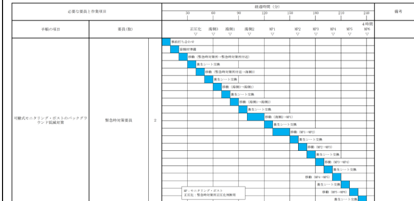
第 1.17-12 図 モニタリング・ポストのバックグラウンド低減対策のタイムチャート
