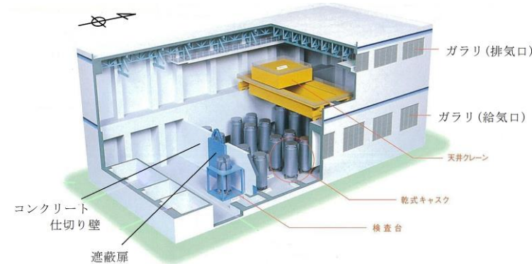
第2-1図 貯蔵建屋鳥瞰図
