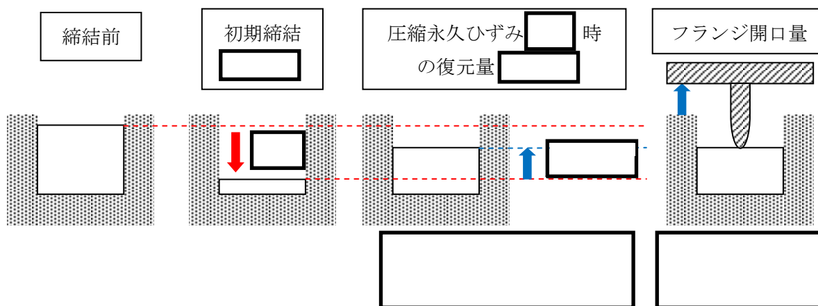
第6図 圧縮永久ひずみ [redacted] 時のシール材復元量とフランジ開口量
