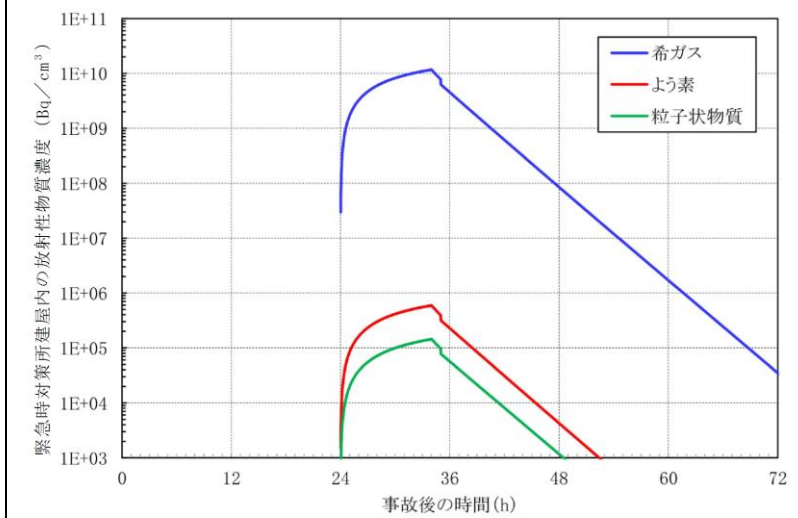
第1-7-1図 緊急時対策所建屋内 (浄化エリア) の放射性物質濃度の推移
