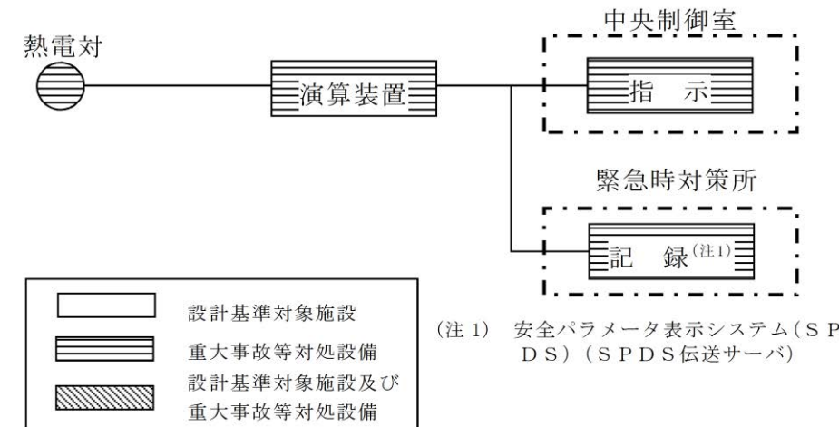
第58-6-23図 ドライウエル温度 (SA)の概略構成図
