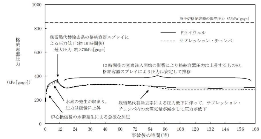
第58-8-28図 格納容器破損モード「水素燃焼」における格納容器圧力の推移
