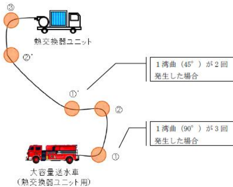
図 20 想定される消防ホースの引き回しパターン (イメージ)
