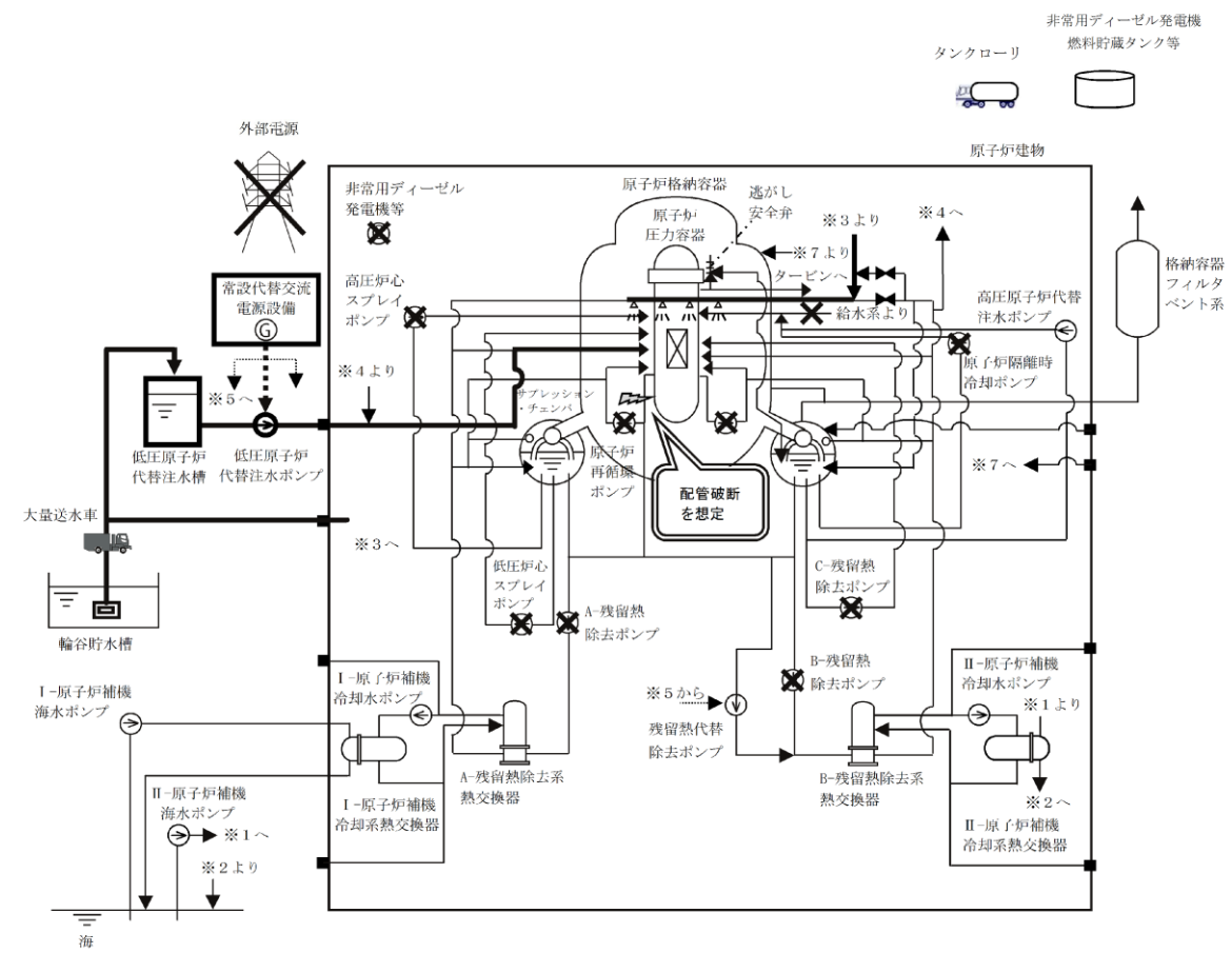
図1 重大事故等対策概要図
