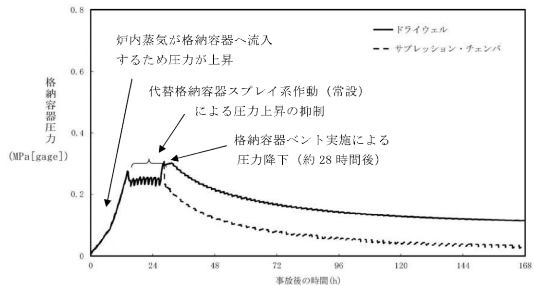
第 4.1.1-3 図 高圧・低圧注水機能喪失時における格納容器圧力の推移
