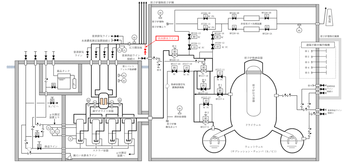
図1 雨水排水ライン系統図
