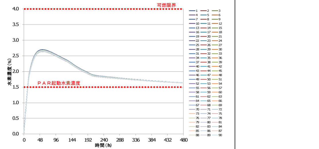
【参考】本文図 2. 2. 2-16 原子炉建物原子炉棟4階の全サブポリウムの水素濃度の時間変化 (設計条件, ベント無し)
