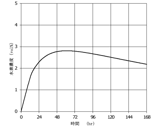
図 2.2.1.2-2 原子炉建物原子炉棟 4 階の水素濃度の時間変化
