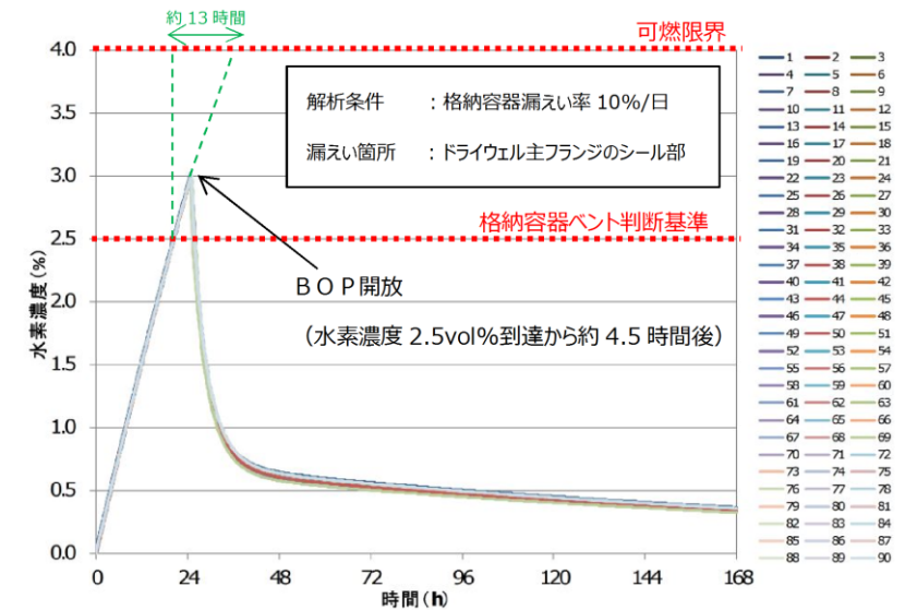
図11 原子炉建物燃料取替階ブローアウトパネル開放による水素濃度の時間変化 (PAR及び格納容器ベント不作動時)
