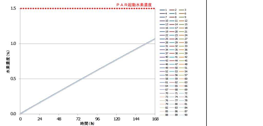
図 2 原子炉建物原子炉棟 4 階のサブボリュームの水素濃度の時間変化 (設計条件, 格納容器漏えい率 0.5%/日)
