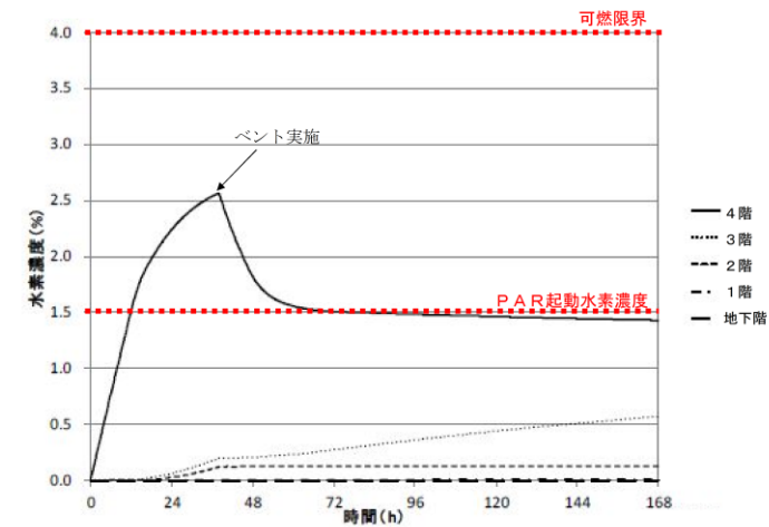
図 2.2.2-17 各フロアの水素濃度の時間変化
