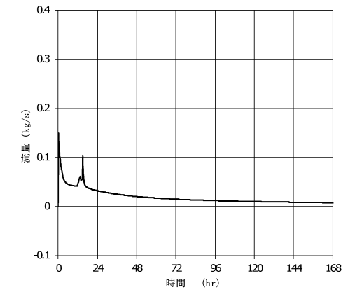
図 2.2.1.2-4 原子炉建物原子炉棟 4 階からのガス流出量の時間変化
