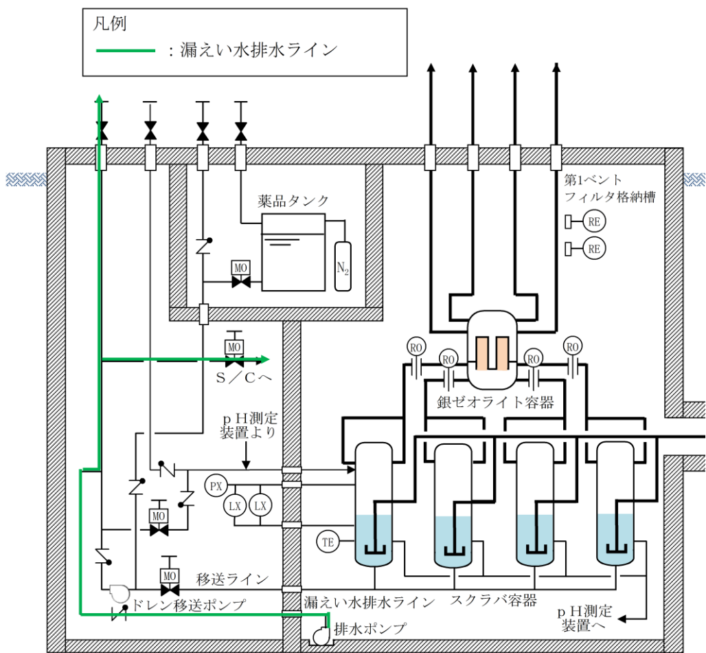
図3 排水設備系統概略図
