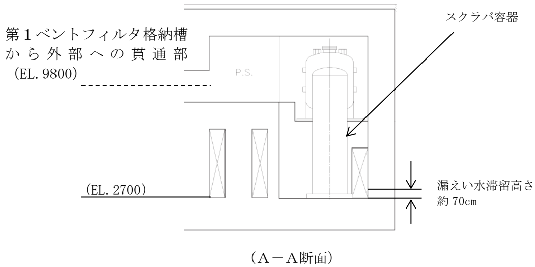
(A-A断面) 図4 第1ベントフィルタ格納槽から外部への貫通部と 漏れい水の高さの関係
