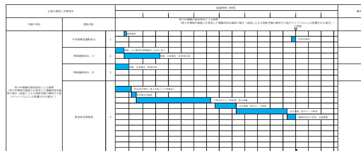
図 3.5-4 原子炉補機代替冷却系による補機冷却水確保タイムチャート*
