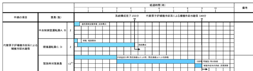
図 3.5-2 代替原子炉補機冷却系による補機冷却水確保タイムチャート*
