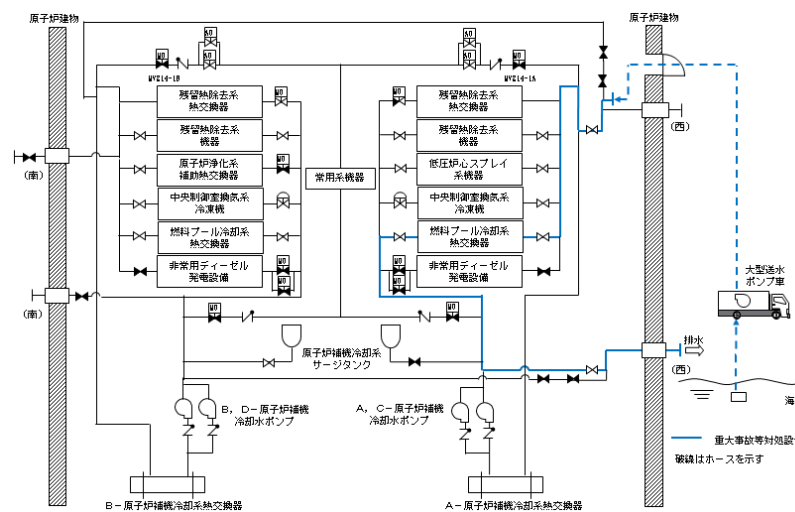
図 3.11-10 原子炉補機代替冷却系 系統概要図
