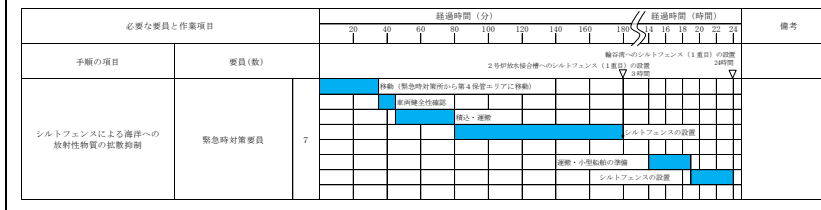
図 3.12-6 海洋への放射性物質の拡散抑制 (シルトフェンス) のタイムチャート※
