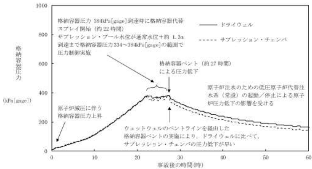
感度解析（サブプレッション・チェンバスプレイ実施）
