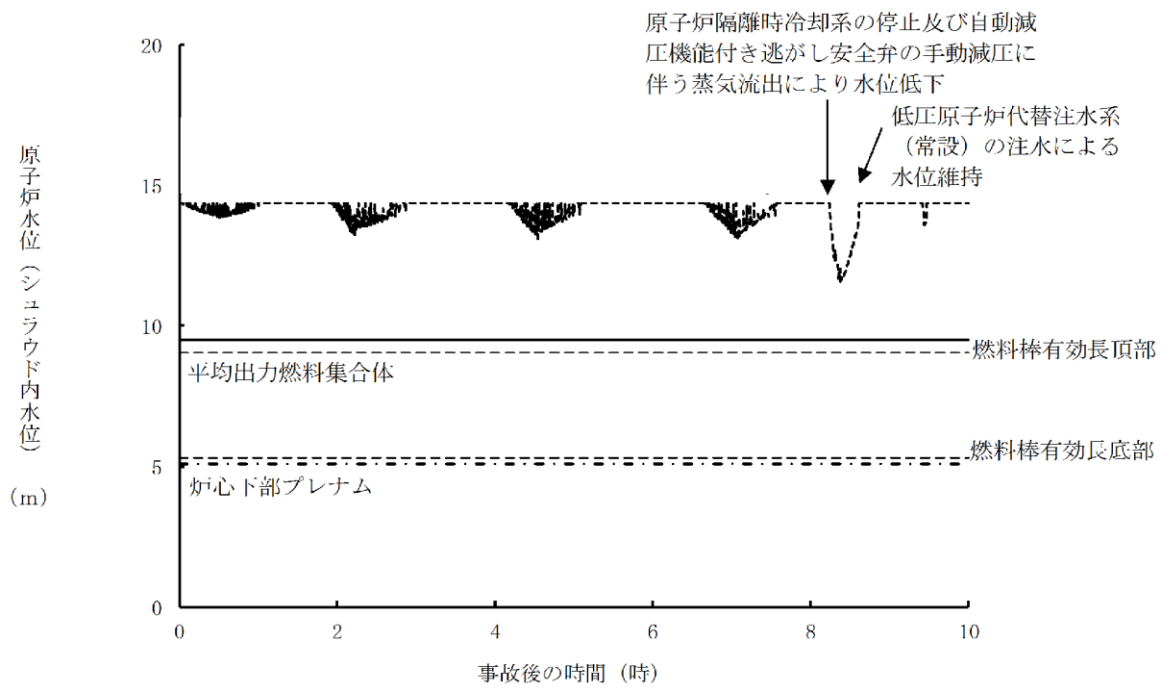
図2 減圧時の原子炉水位 (シュラウド内)
