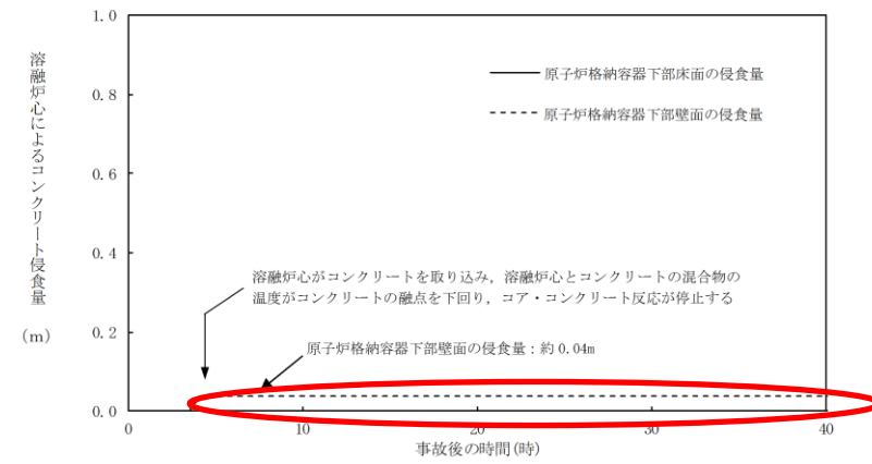
図1 原子炉格納容器下部床面及び壁面のコンクリート侵食量の推移 (溶融炉心の崩壊熱を保守的に考慮する場合)
