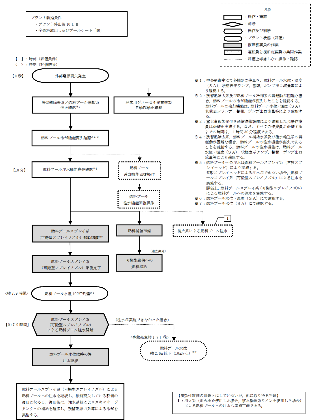
第 4.1.1-2 図 「想定事故 1」の対応手順の概要
