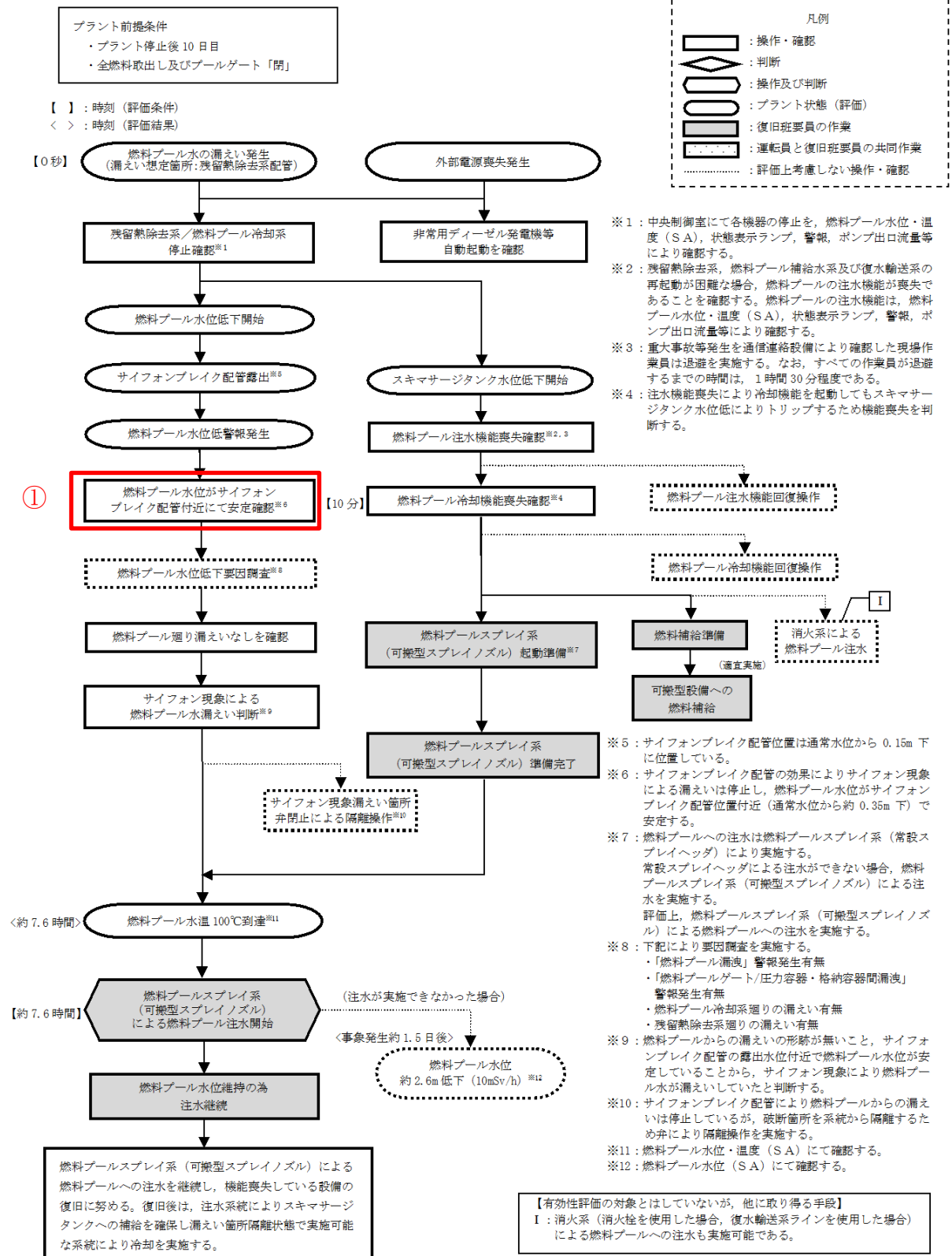
第 4.2.1-2 図 「想定事故 2」の対応手順の概要
