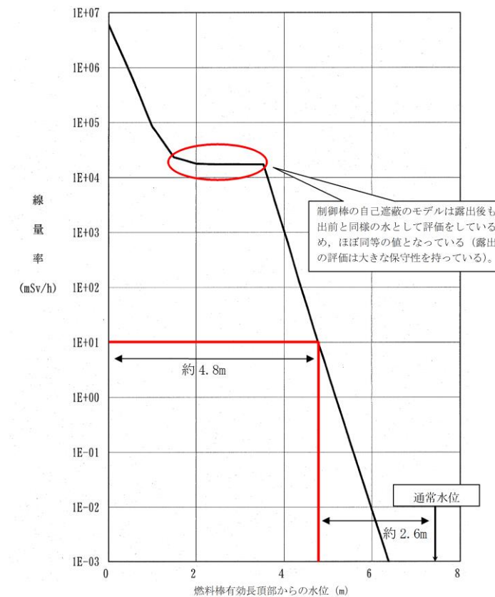
図7 放射線の遮蔽が維持される水位
