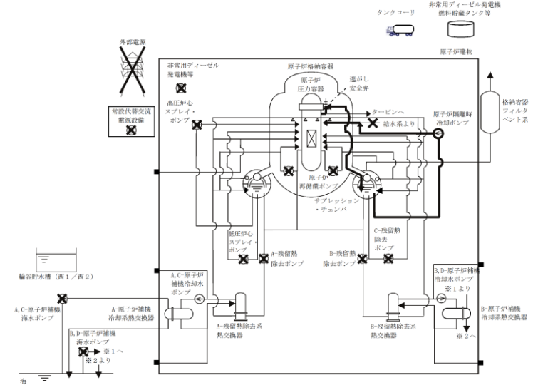
第2.3.1.1-1(1) 図 「全交流動力電源喪失（外部電源喪失+DG失敗）+HPCS失敗」の重大事故等対策の概略系統図 (原子炉注水)
