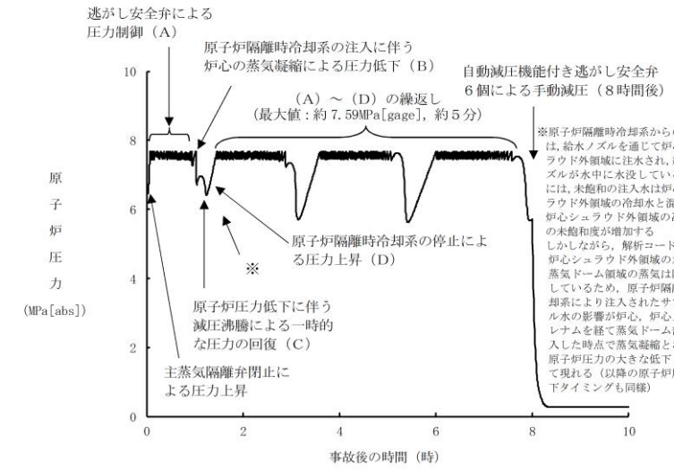
第 2.3.1.2-1(1) 図 原子炉圧力の推移
