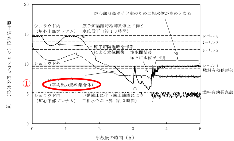
第 2.3.3-6 図 原子炉水位 (シユラウド内外水位) の推移
