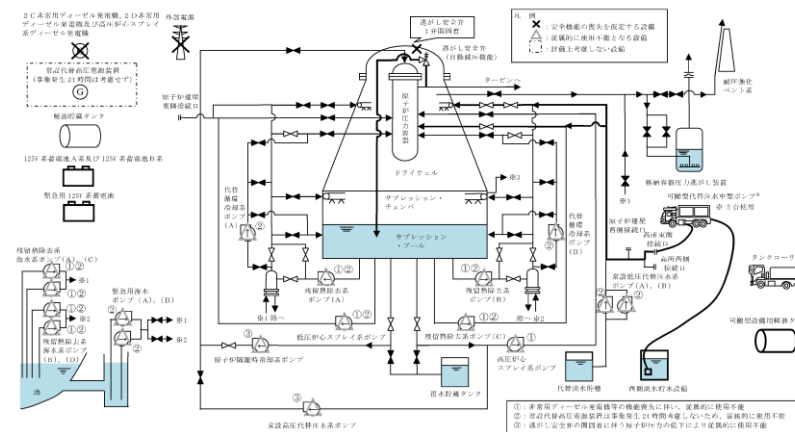
第 2.3.3-1 図 全交流動力電源喪失 (TBP) 時の重大事故等対策の概略系統図 (2/3) (低压代替注水系 (可搬型) による原子炉注水及び代替格納容器スプレィ冷却系 (可搬型) による格納容器冷却段階)
