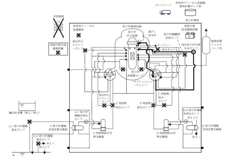
第 2.3.2.1-1(1) 図 「全交流動力電源喪失 (外部電源喪失+DG 失敗) +高圧炉心冷却失敗」の重大事故等対策の概略系統図 (原子炉注水)
