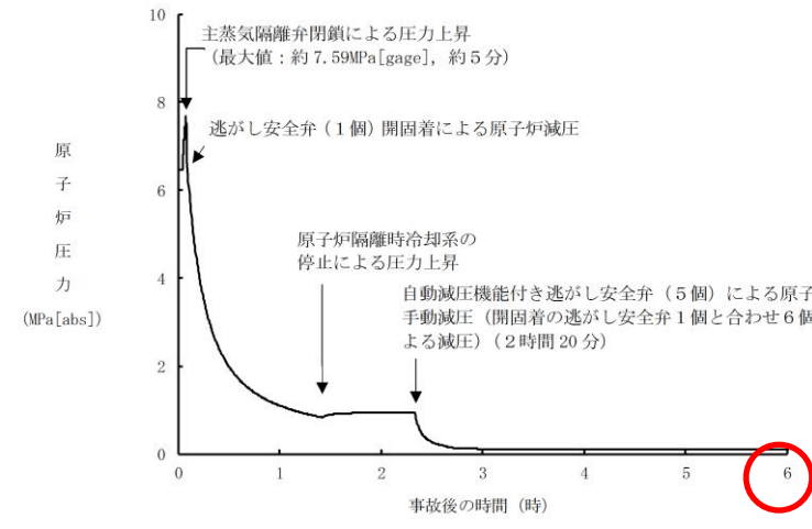
第2.3.4.2-1(1) 図 原子炉圧力の推移
