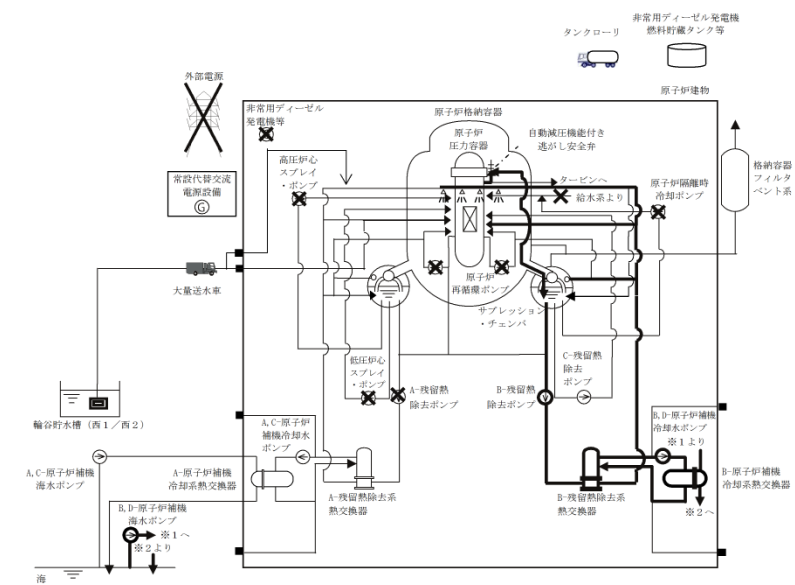
第 2.3.4.1-1(3) 図 「全交流動力電源喪失 (外部電源喪失+DG 喪失)+SRV 再閉失敗+HPCS 失敗」の重大事故等対策の概略系統図 (原子炉注水及び原子炉格納容器除熱)
