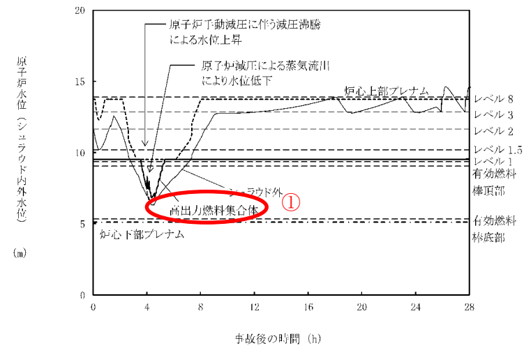
第 2.3.4.9 図 原子炉水位 (シユラウド内外水位) の推移
