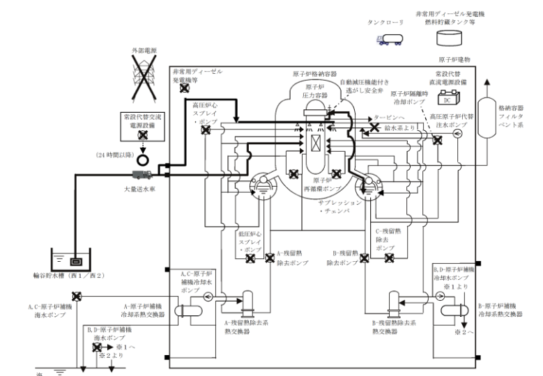
第 2.3.2.1-1(2) 図 「全交流動力電源喪失 (外部電源喪失+DG 失敗) +高圧炉心冷却失敗」の重大事故等対策の概略系統図 (原子炉減圧, 原子炉注水及び原子炉格納容器冷却)
