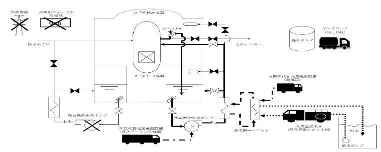
第 2.3.4.4 図 「全交流動力電源喪失 (外部電源喪失+DG 喪失)+SRV 再閉失敗」の重大事故等対策の概略系統図 (4/4) (原子炉注水及び原子炉格納容器除熱)
