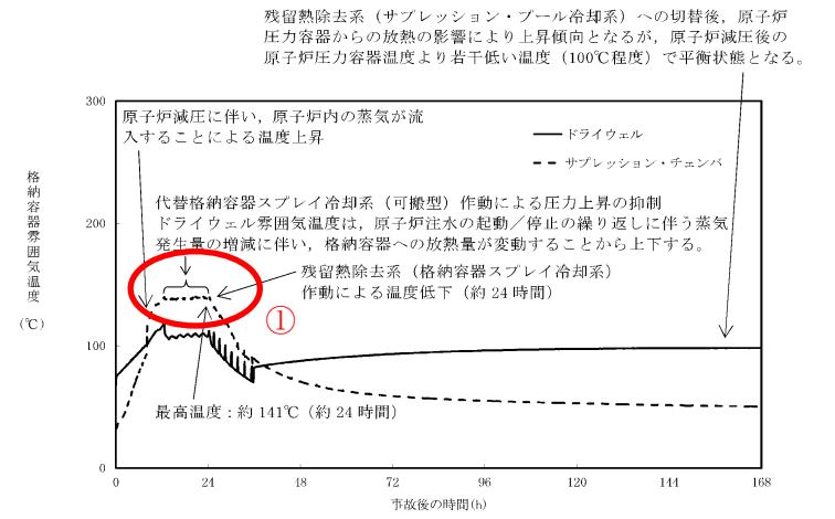
第 2.3.2-14 図 格納容器雰囲気温度の推移
