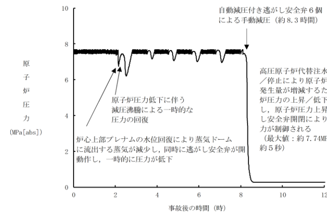
第 2.3.2.2-1(1) 図 原子炉圧力の推移
