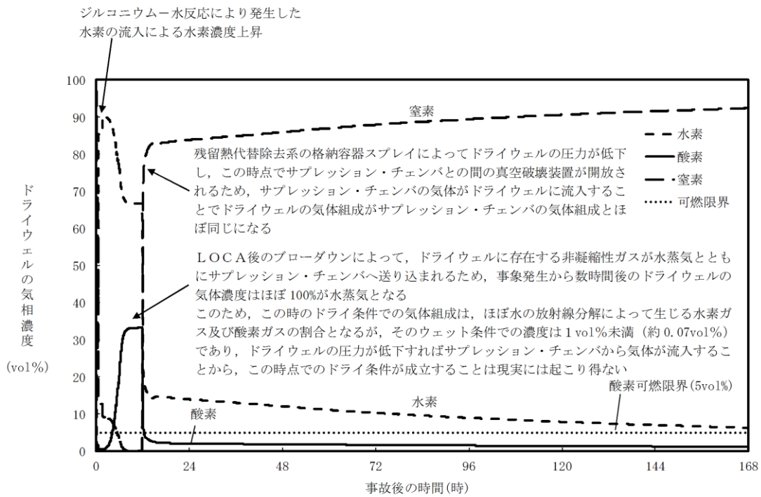
第 3. 4. 2-1 (5) 図 ドライウエルの気相濃度の推移 (ドライ条件)
