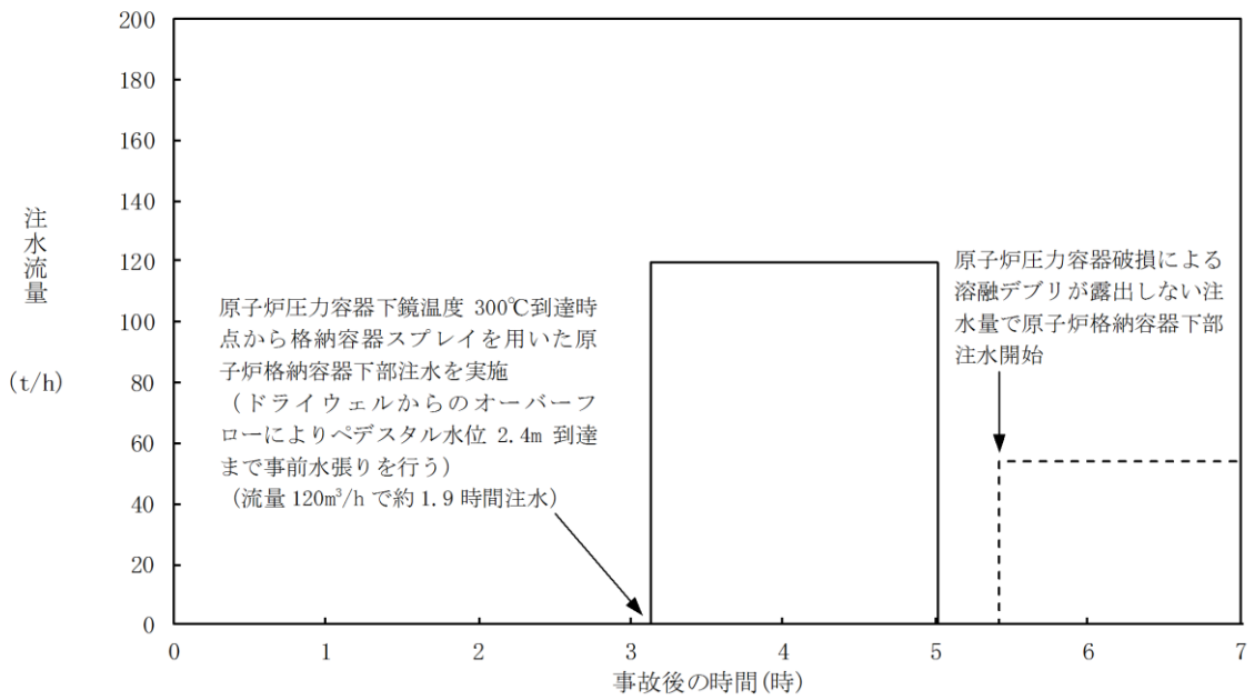
第 3. 3. 2-1 (6) 図 注水流量の推移
