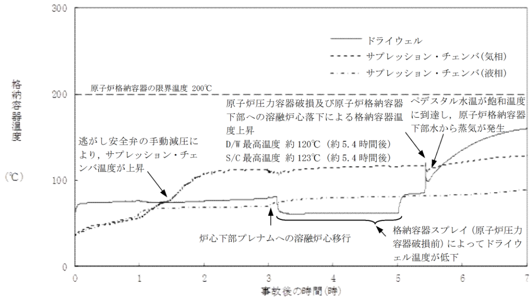
第 3. 3. 2-1 (4) 図 格納容器温度の推移
