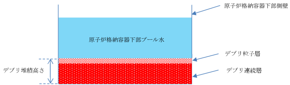
図1 デブリ堆積高さの概念図
