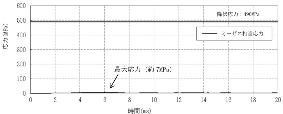
図7 水蒸気爆発による原子炉格納容器下部外側鋼板の応力の変化 (約 3.8m, 現実的な想定) ※1
