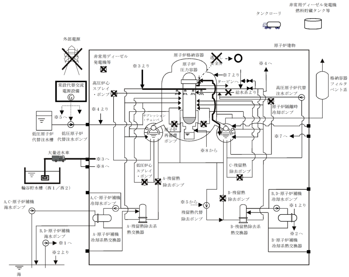
第 3.2.1-1(2) 図 「高圧溶融物放出／格納容器雰囲気直接加熱」の重大事故等対策の概略系統図 (原子炉压力容器破損前の原子炉減圧, 原子炉格納容器下部注水)
