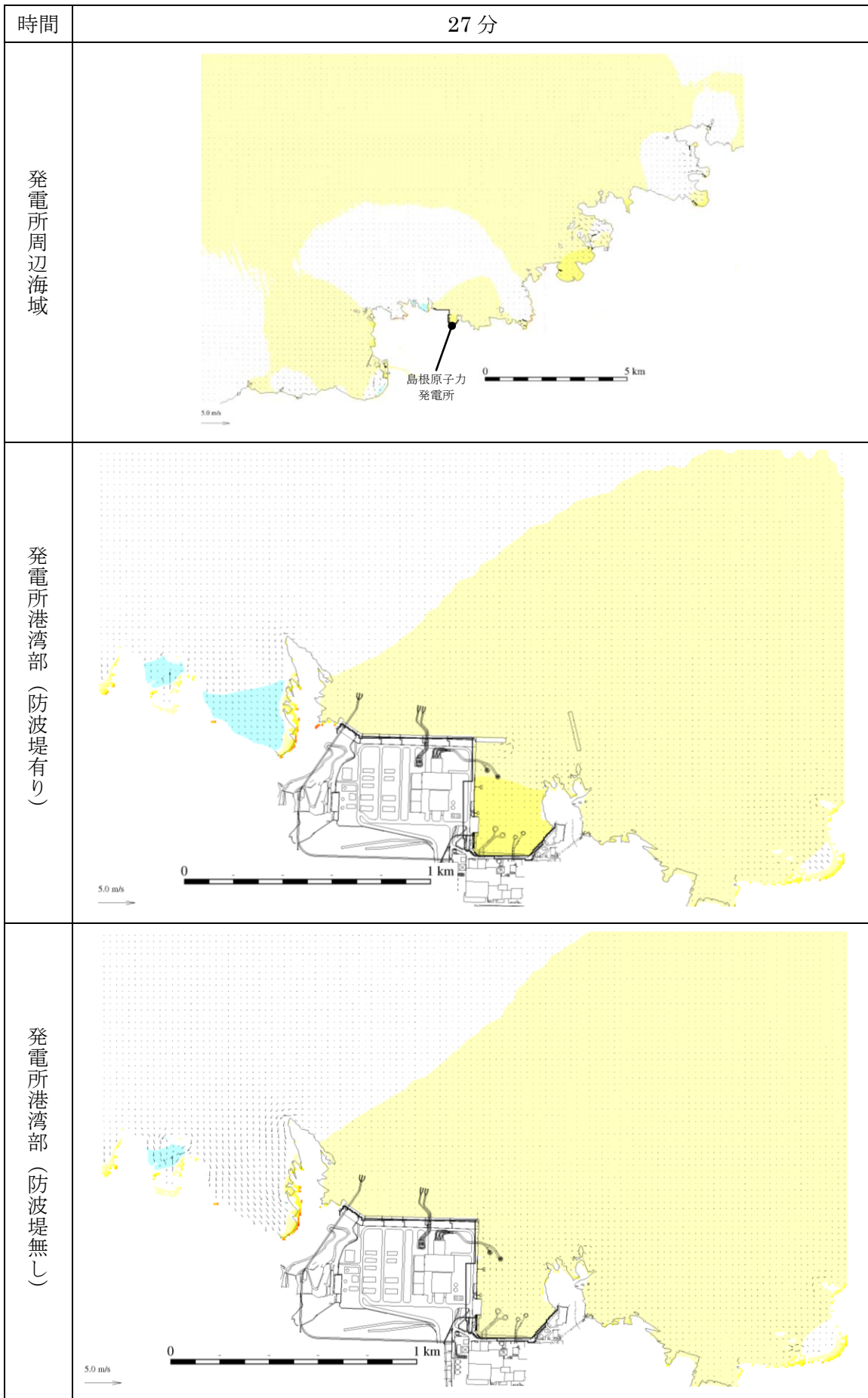
第 4 図 (55) 基準津波 4 の水位変動・流向ベクトル
