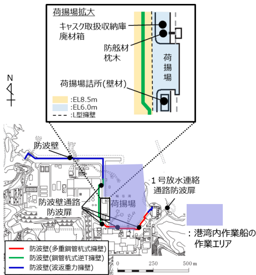
港湾内に面する津波防護施設に考慮する 漂流物の配置
