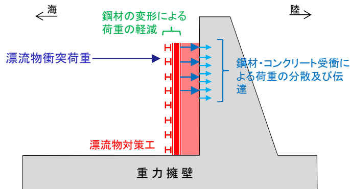
漂流物対策工における荷重図
