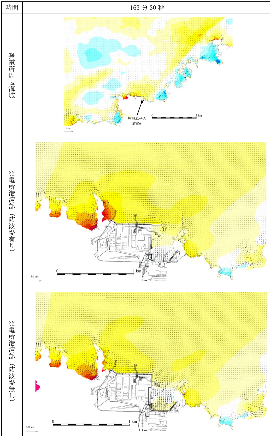
第 1 図(128) 基準津波 1 の水位変動・流向ベクトル
