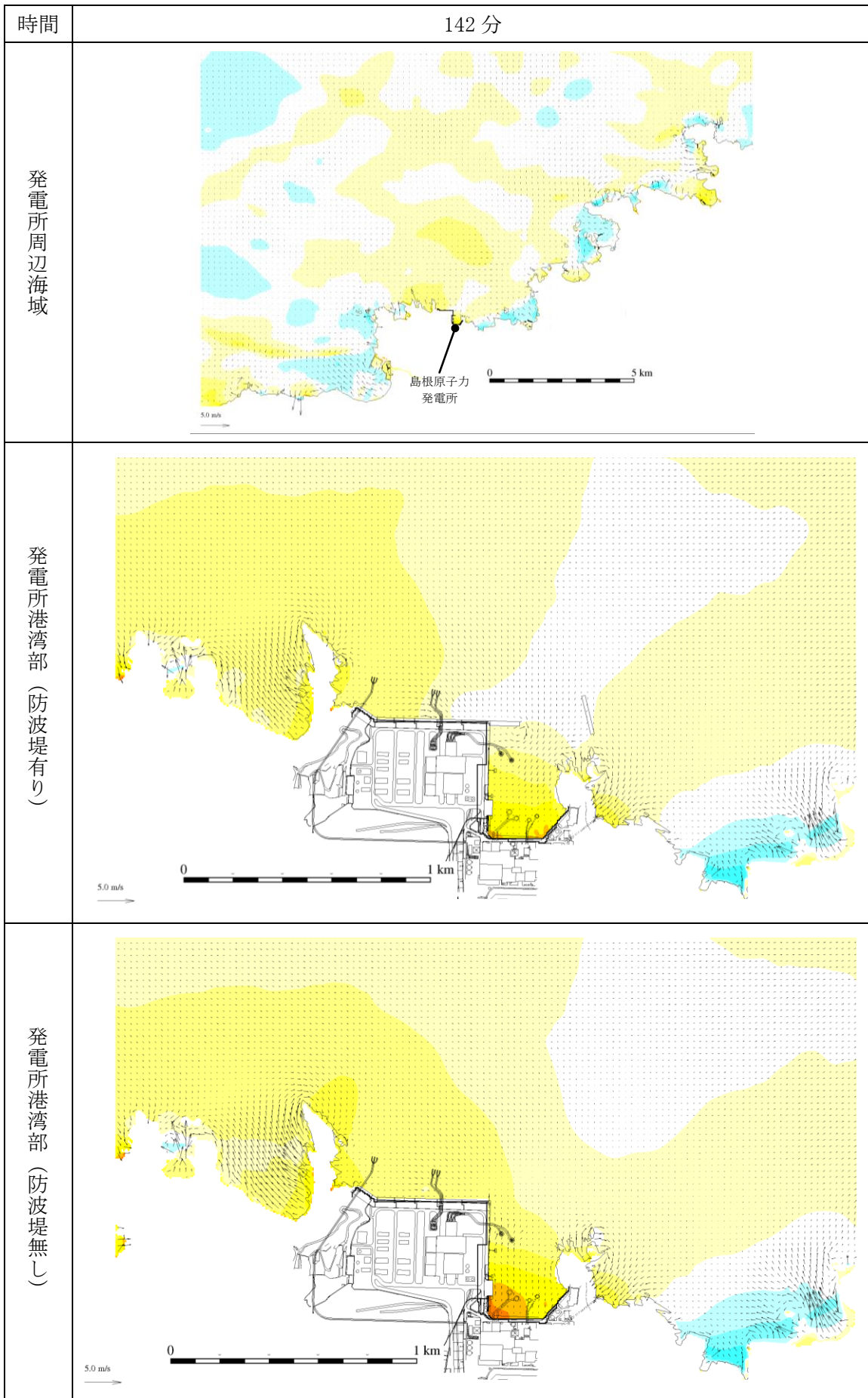
第 1 図(85) 基準津波 1 の水位変動・流向ベクトル
