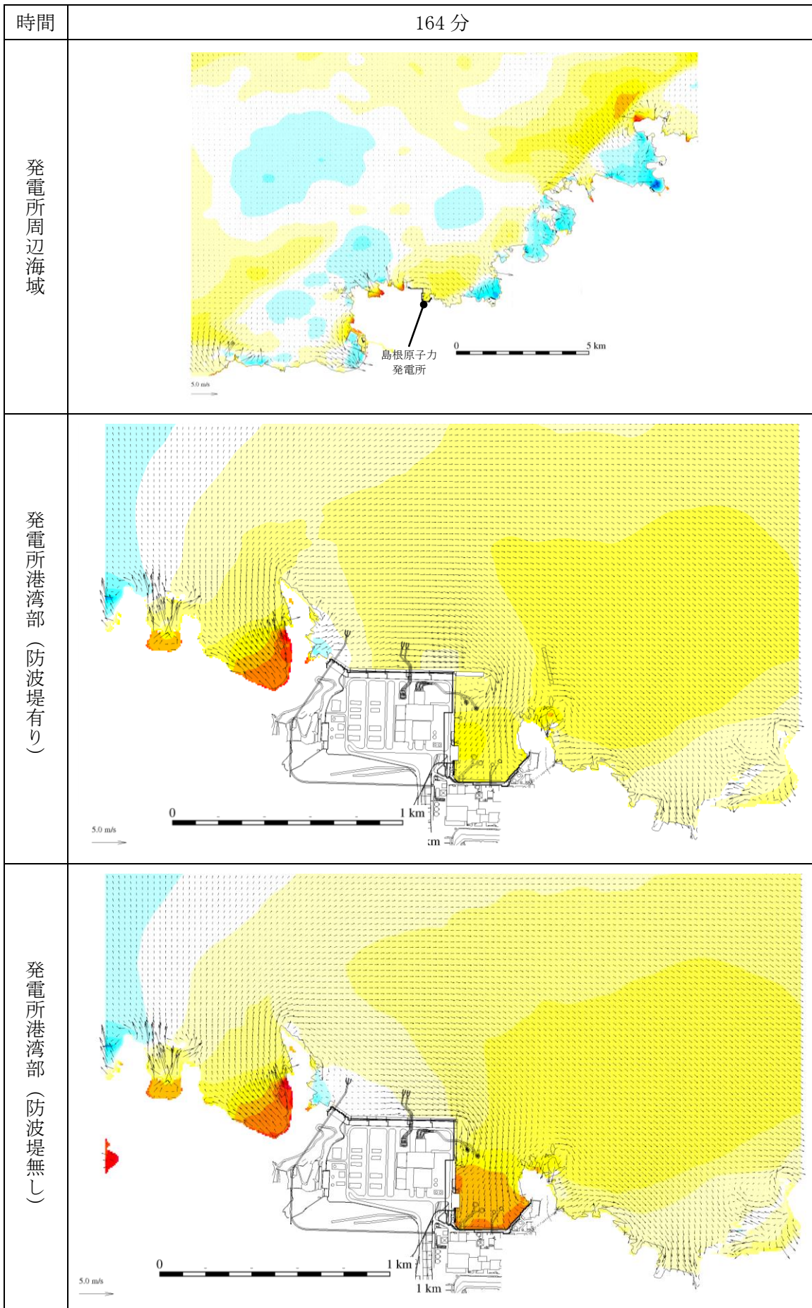
第 1 図(129) 基準津波 1 の水位変動・流向ベクトル
