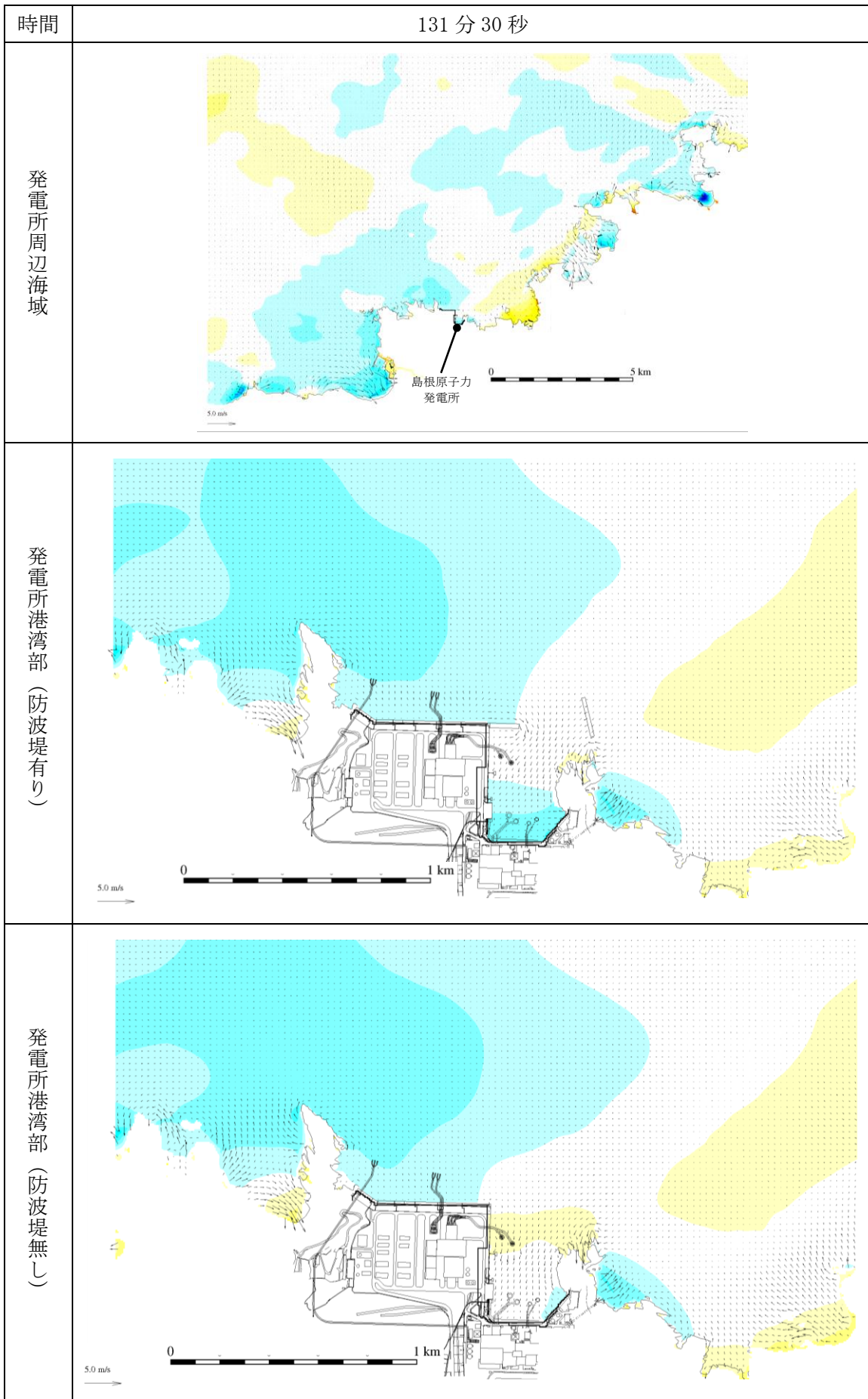
第 1 図(64) 基準津波 1 の水位変動・流向ベクトル
