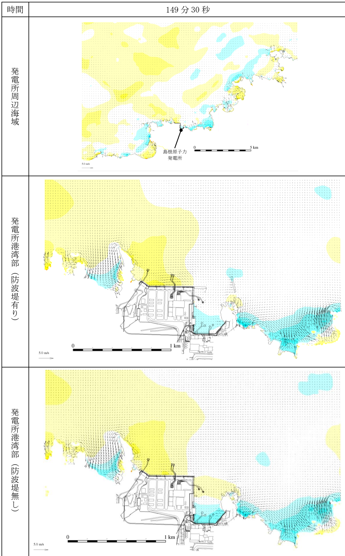
第 1 図(100) 基準津波 1 の水位変動・流向ベクトル
