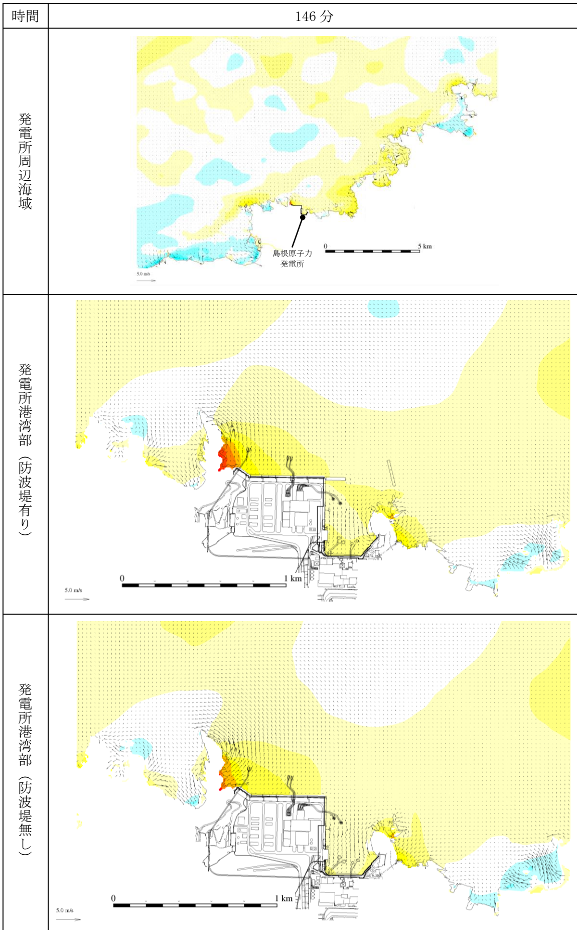
第 1 図(93) 基準津波 1 の水位変動・流向ベクトル
