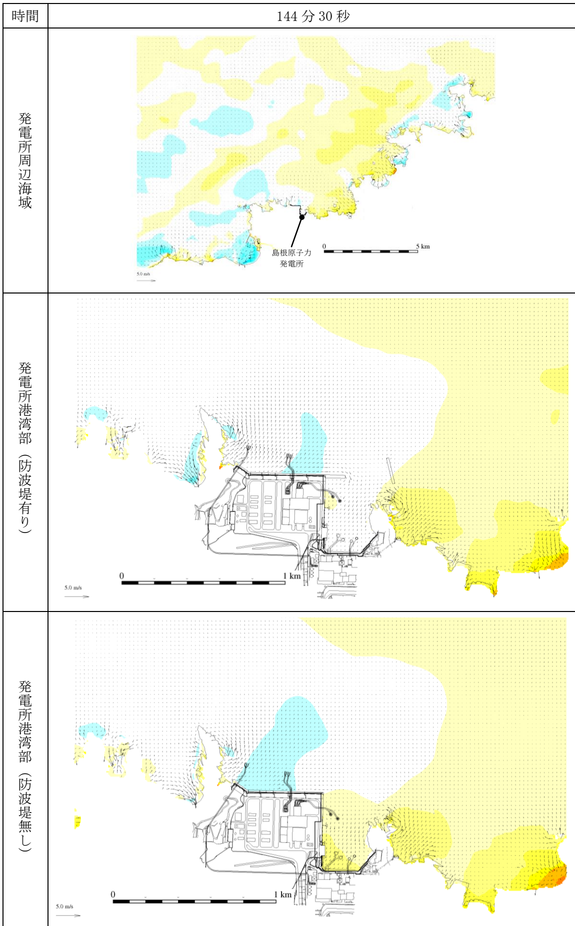
第 1 図(90) 基準津波 1 の水位変動・流向ベクトル
