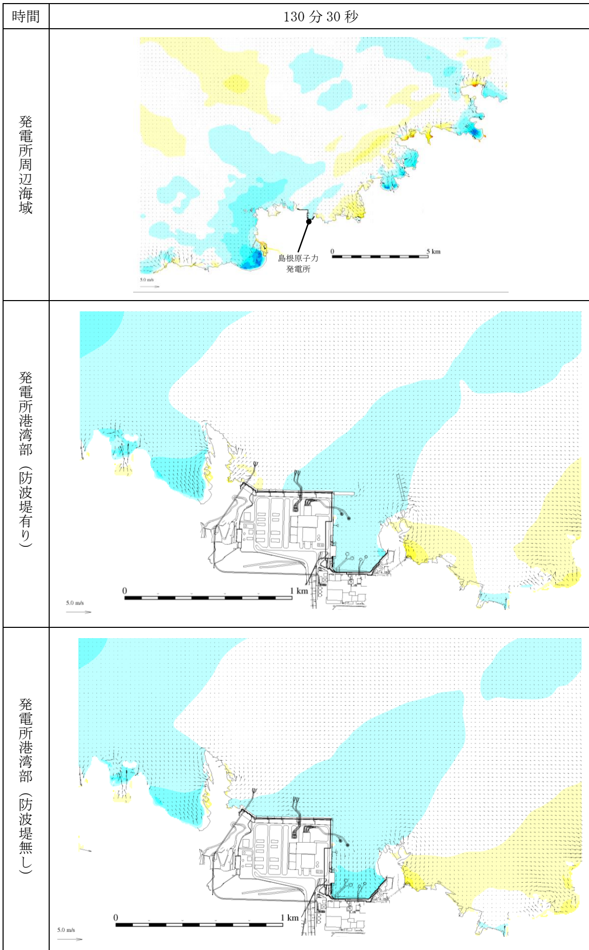
第 1 図(62) 基準津波 1 の水位変動・流向ベクトル
