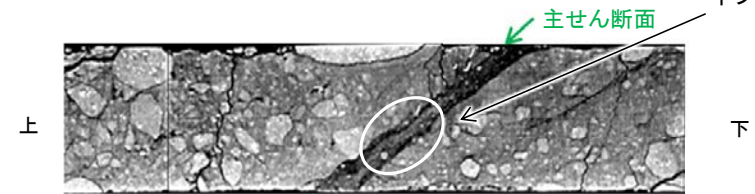
CT画像(H-0.2-75孔)
