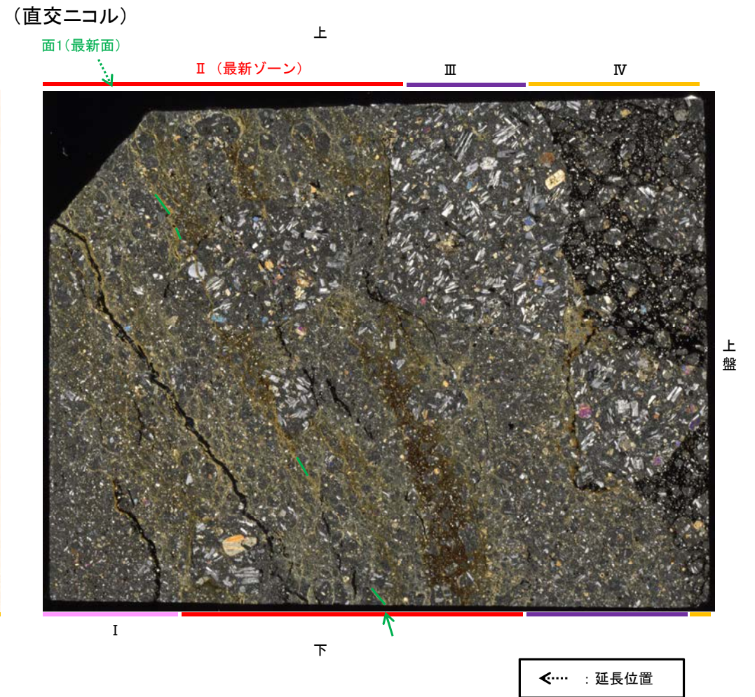
観察用薄片写真(M-2.2_90R)
