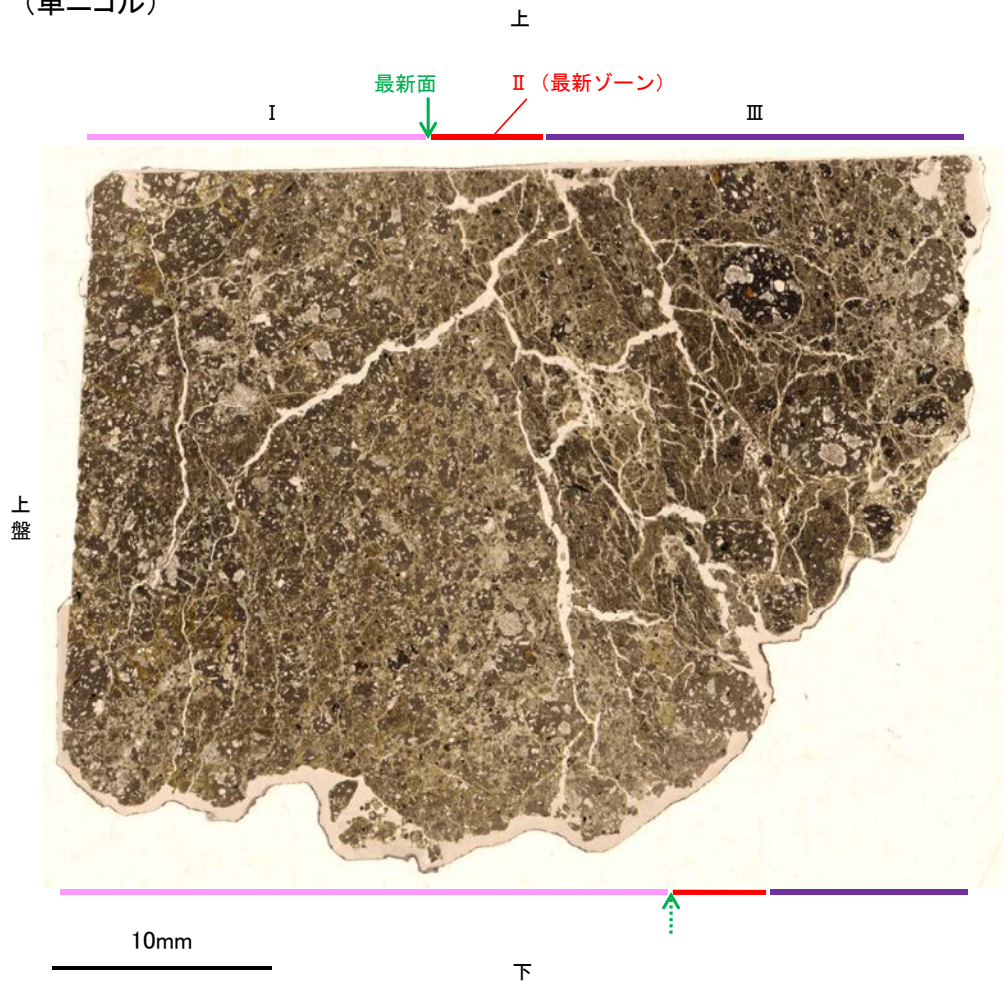
観察用薄片①写真(H-0.2-75_34R)
