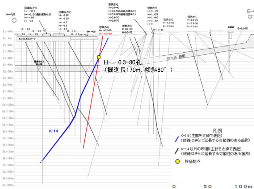
①-①' 断面図
