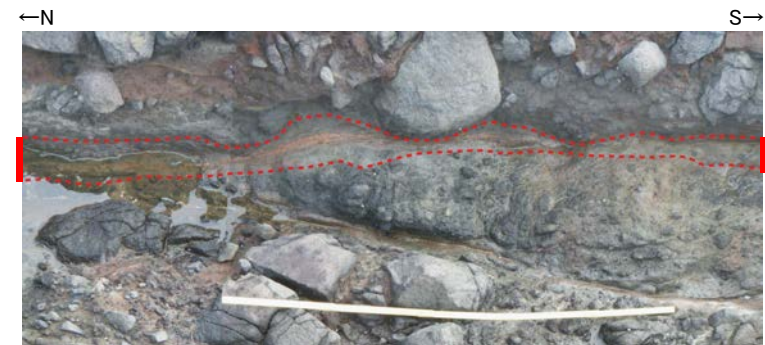
c地点 破砕部の状況写真
