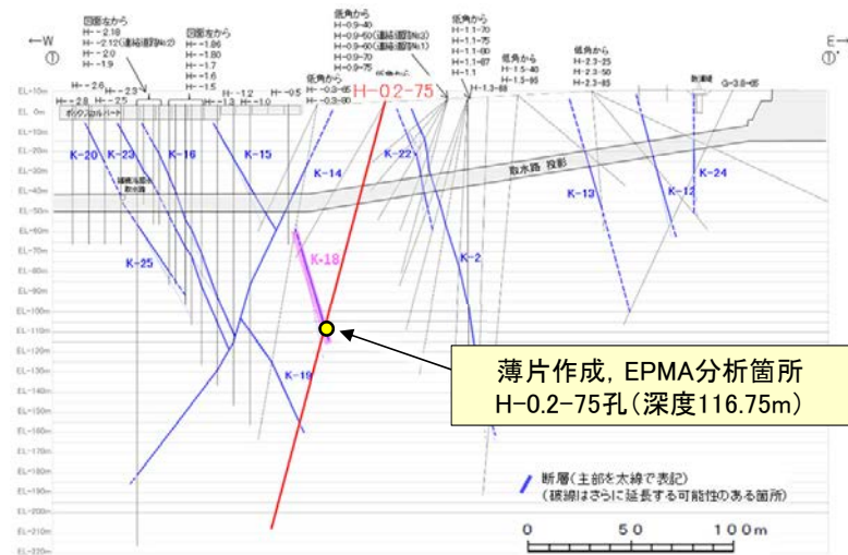
調査位置図(断面図)
