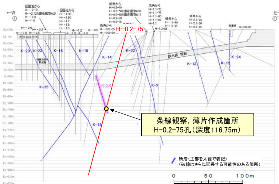
①-①' 断面図
