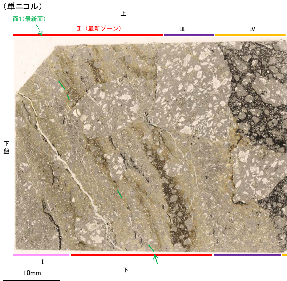
観察用薄片写真(M-2.2_90R)
