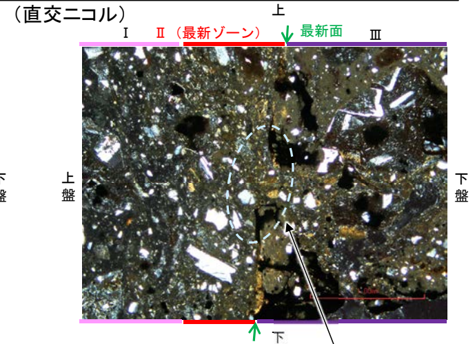
詳細観察範囲写真
