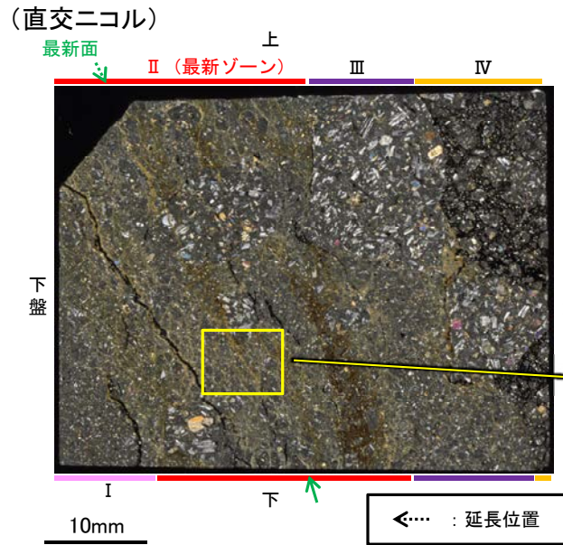
観察用薄片写真(M-2.2_90R)
