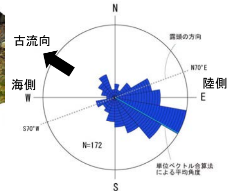
礫のインブリケーションの傾斜方向。傾斜方向の反対向きが古流向を示す。(径5cm以上、傾斜10～50°の礫をグラフ化)
