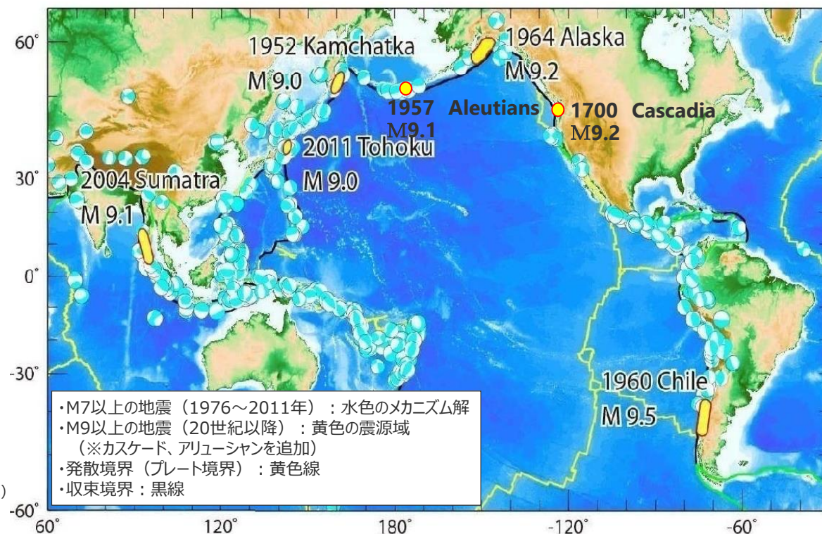
Global CMT による M \geq 7 の地震 (佐竹 (2012) を基に作成)
