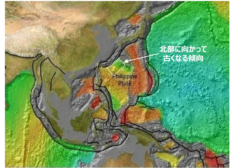
新しい 古い million years 0 20 40 60 80 100 120 140 160 180 200 220 240 260 280
