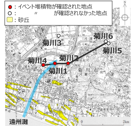
5万分の1地形図「御前崎」(掛川) (国土地理院) に加筆
