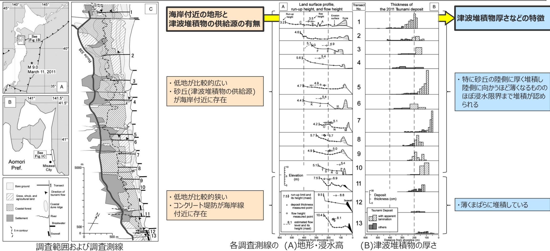
三沢海岸における東北沖地震による浸水深と津波堆積物の厚さの調査結果 (Nakamura et al. (2012)を基に作成)
