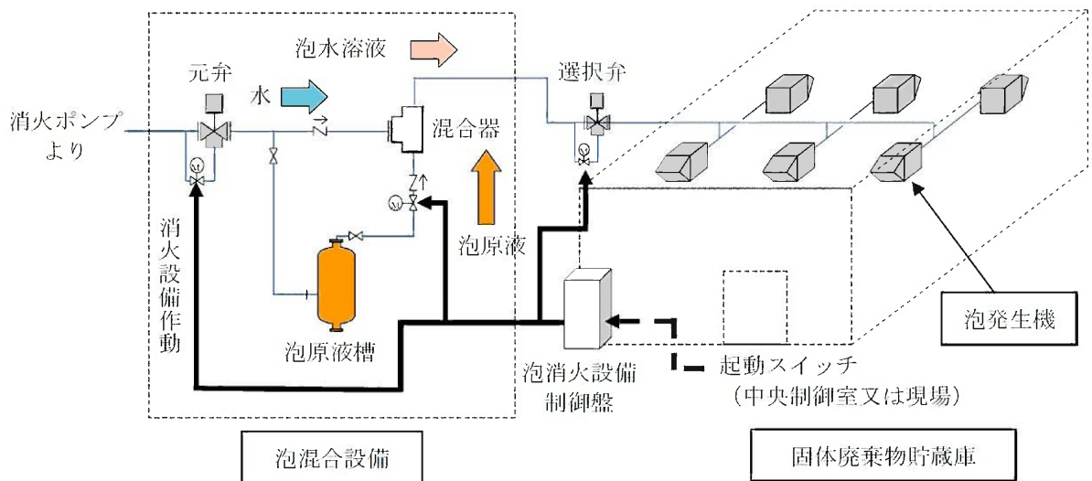
第 10.5.6 図 泡消火設備概要図
