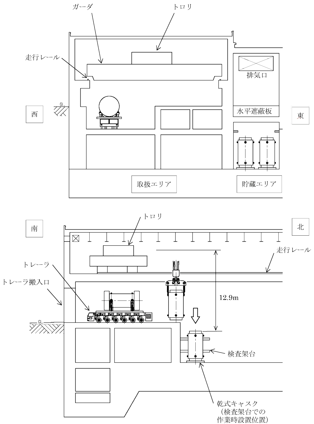
(b) 断面図
