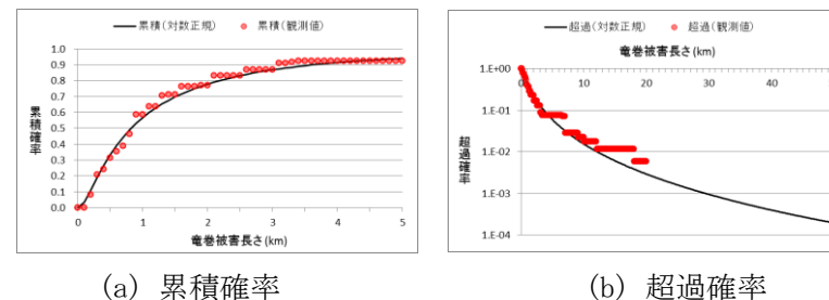
図 2.3.9 竜巻被害長さの確率分布の推定結果と観測値との比較
