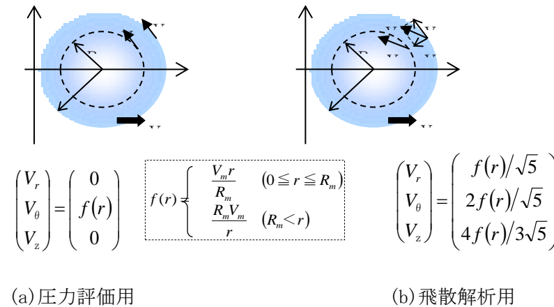
第2.2-1図 ランキン渦モデル
