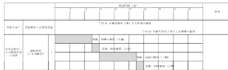
第 1.16-3 図 中央制御室の照明の確保のタイムチャート
