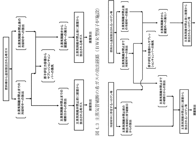
図 4.4 主蒸気管破断のハロゲン等の放出経路 (BWR 型原子炉施設)
