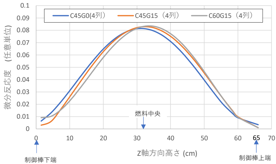
図 A-12 2分割炉心の制御棒微分反応度曲線（曲線の積分値が1となるように規格化） （C45G0（4列）炉心、C45G15（4列）炉心、C60G15（4列）炉心）
