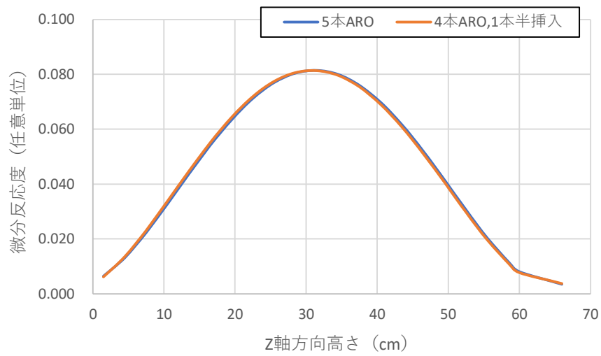
図 A-14 C45G0(4列)炉心のC2制御棒微分反応度曲線 (曲線の積分値が1となるように規格化) (青線：C2以外の5本の制御棒は全引抜き、 オレンジ線：C2と反対側のS5制御棒を半分まで挿入)
