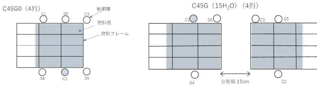
図 A-13 C45G0(4 列)炉心 C45G0(4 列)炉心の配置図
