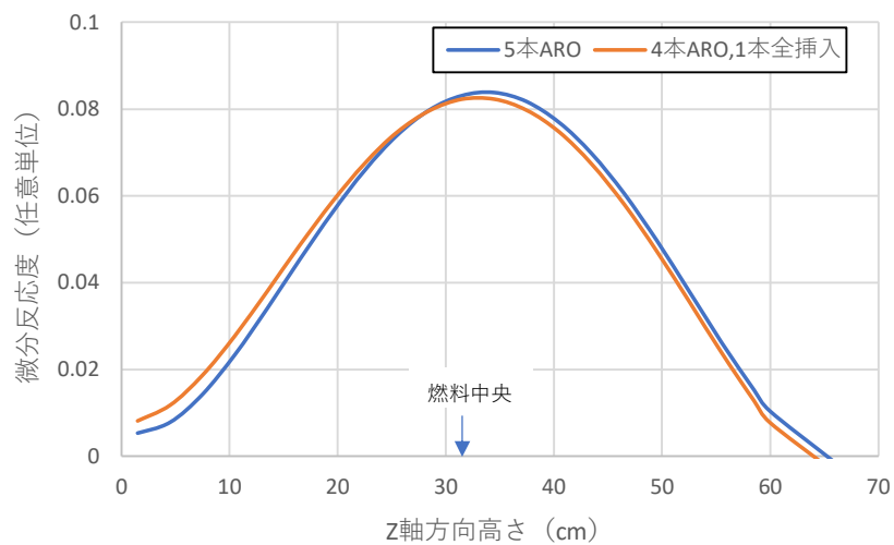
図 A-15 C45G15(4列)炉心のC2制御棒微分反応度曲線 (曲線の積分値が1となるように規格化) (青線：C2以外の5本の制御棒は全引抜き、 オレンジ線：C2と反対側のS5制御棒を半分まで挿入)
