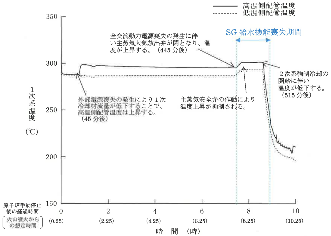
第6図 1次系温度 (高温側、低温側)
