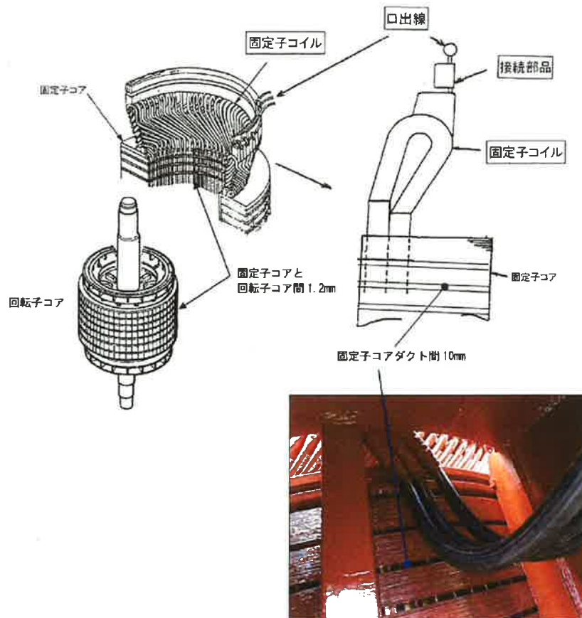
図6 海水ポンプモータの内部構造
