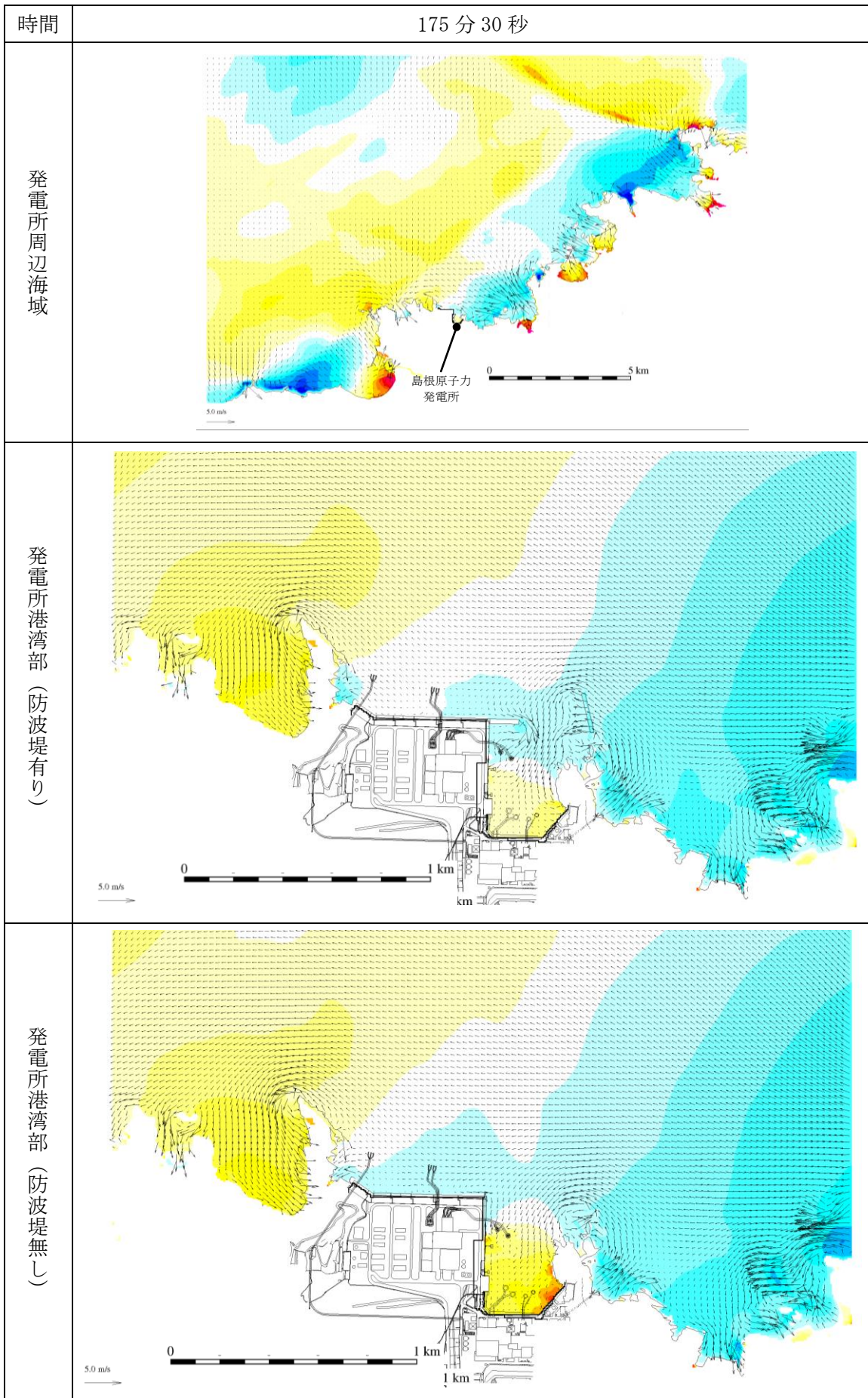
第 1 図(152) 基準津波 1 の水位変動・流向ベクトル
