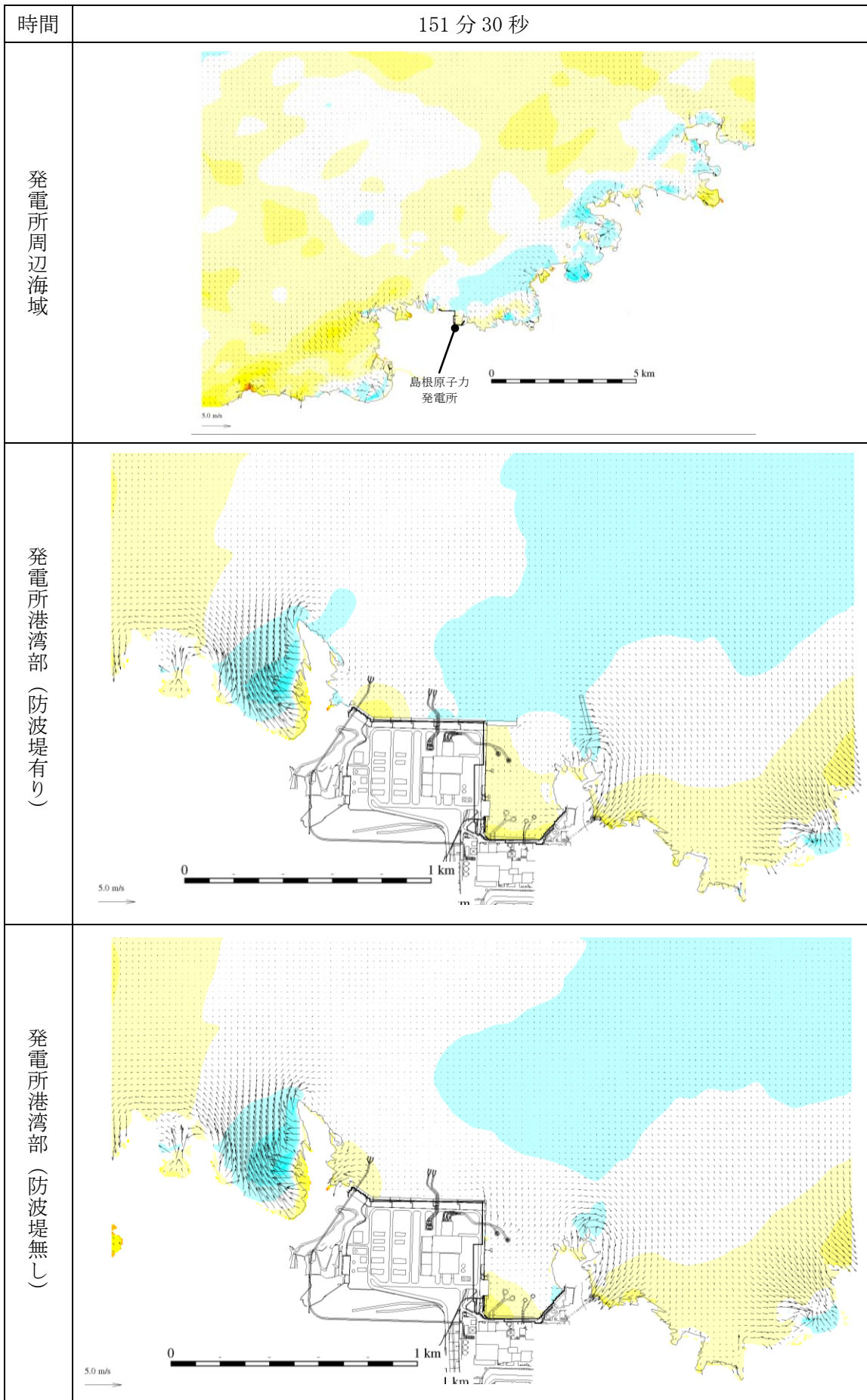
第 1 図(104) 基準津波 1 の水位変動・流向ベクトル
