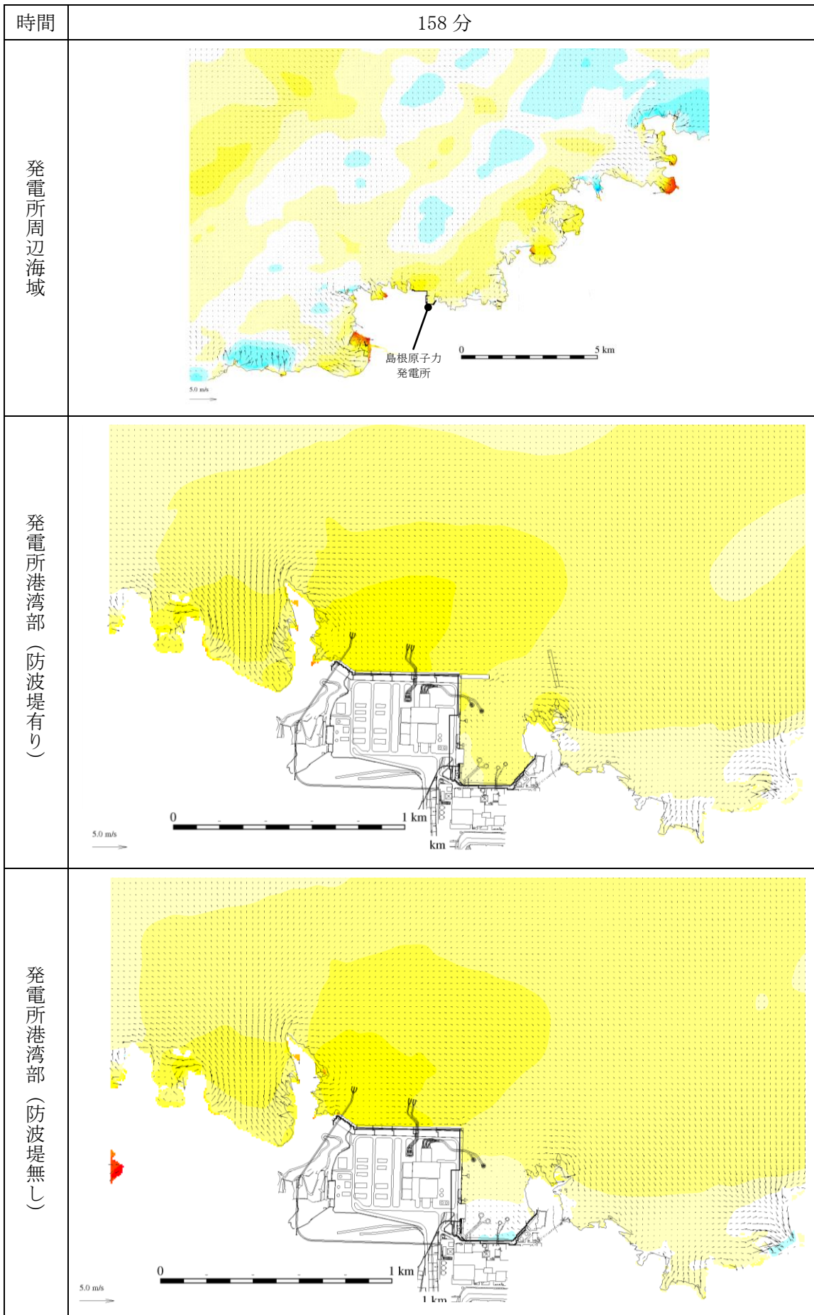
第 1 図(117) 基準津波 1 の水位変動・流向ベクトル
