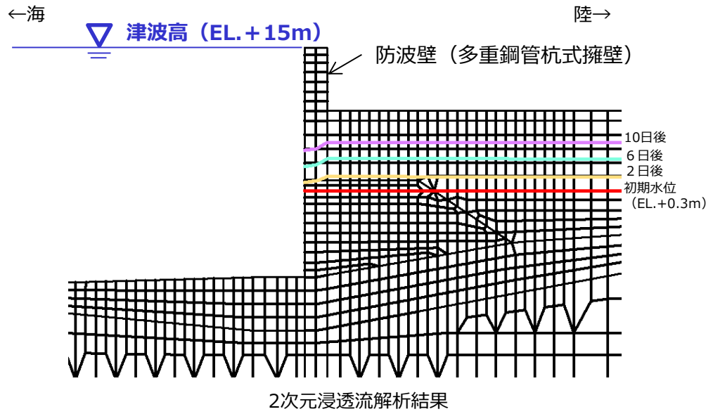
第 5-45 図 2次元浸透流解析結果 (②-②断面)
