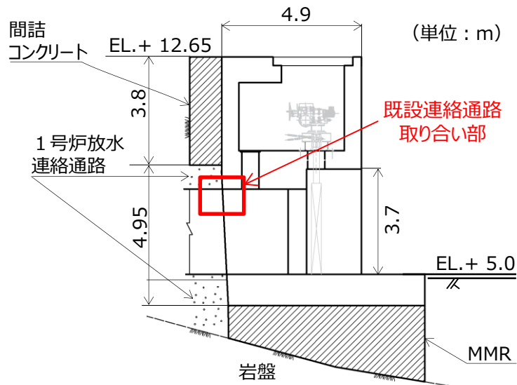
第 8-28 図 1 号放水連絡通路防波扉 A-A 断面図
