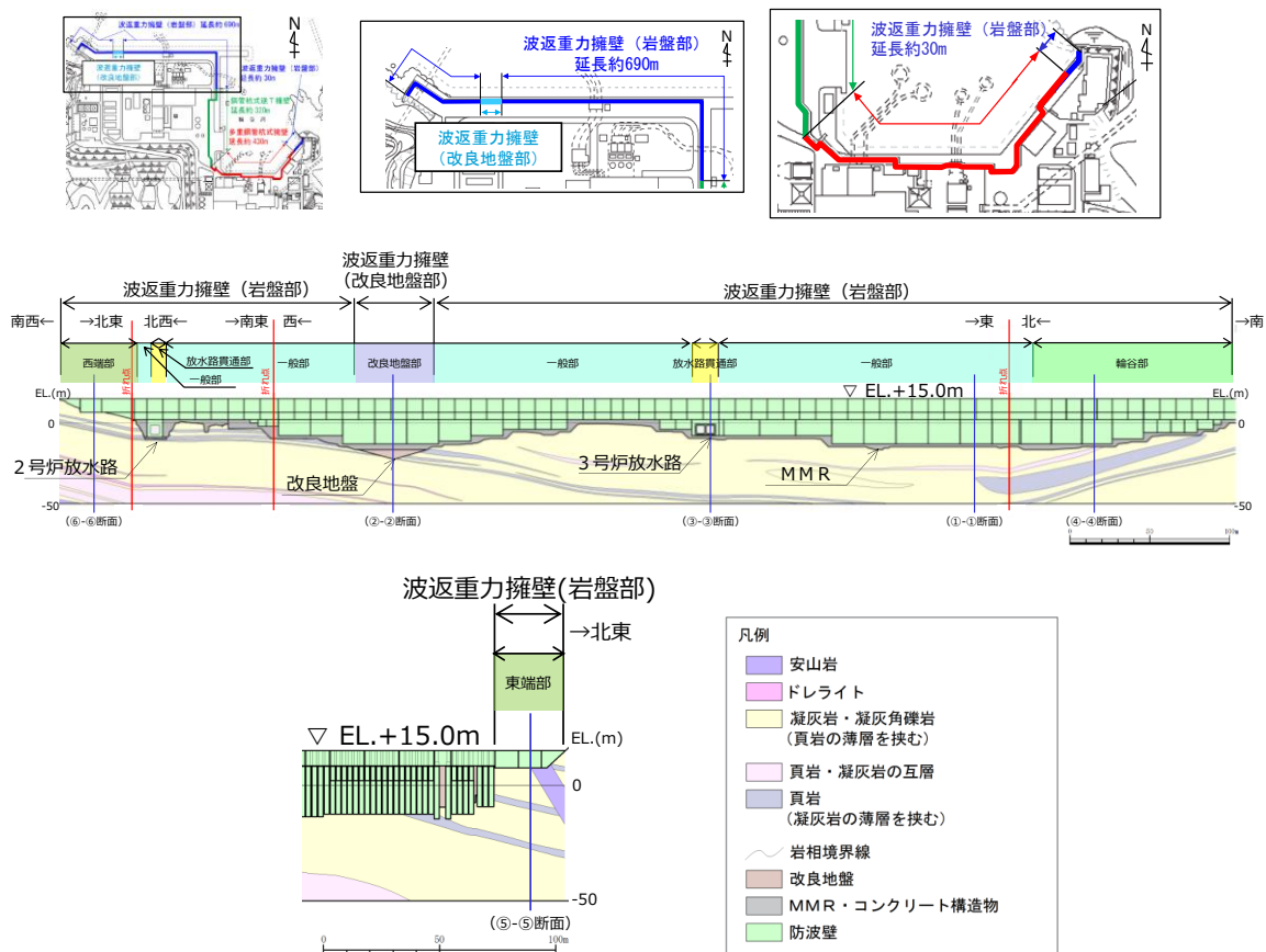
第 7-11 図 防波壁（波返重力擁壁）の地質縦断図
