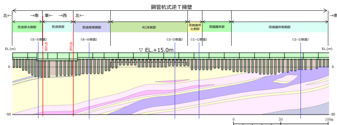
第 6-10 図 防波壁（鋼管杭式逆T擁壁）の地質縦断面図
