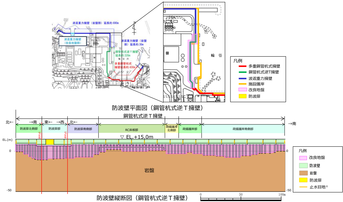
第6-2図 防波壁（鋼管杭式逆T擁壁）縦断面図
