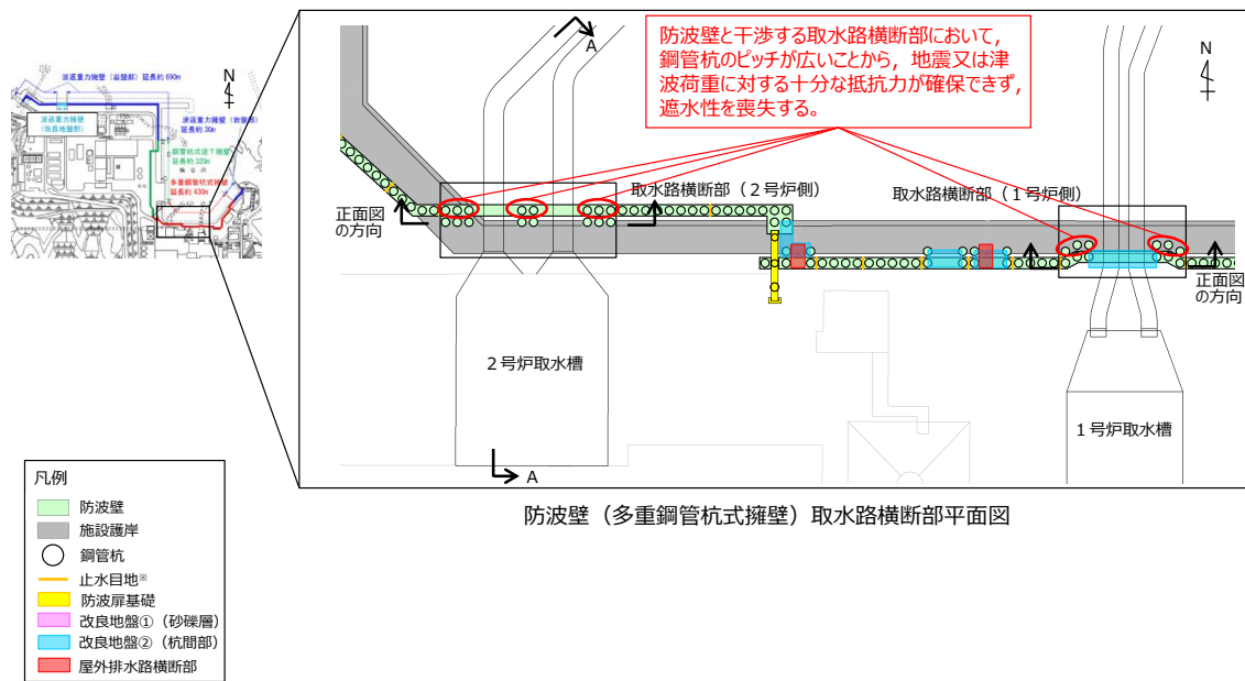
第 5-26 図 防波壁 (多重鋼管杭式擁壁) 弱部②概要図 (取水路横断面)
