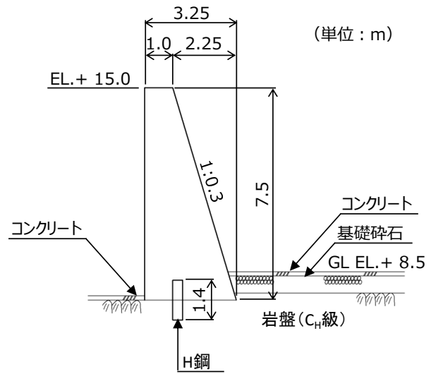
第 7-5(5) 図 防波壁 (波返重力擁壁) 東端部 (⑤-⑤) 断面図
