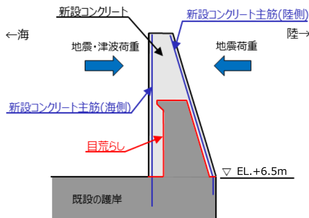
第7-36図 重力擁壁の構造図
