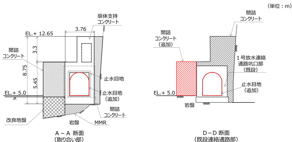
第8-25 図 1号放水連絡通路防波扉の断面図（2）
