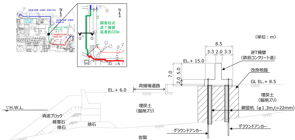
第 6-4(1) 図 防波壁（鋼管杭式逆 T 擁壁）荷揚護岸北側部 (①—①断面) 断面図
