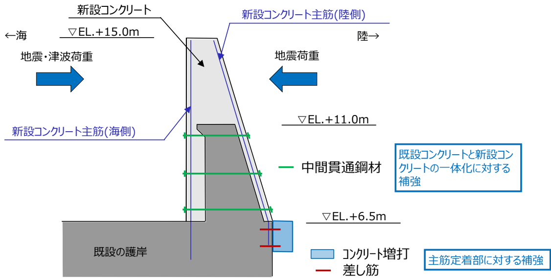
対策工の構造例
