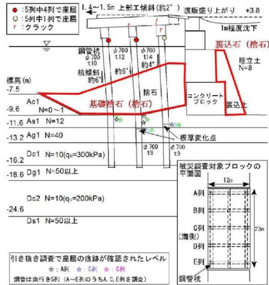
断面図 (神戸港T栈橋)
