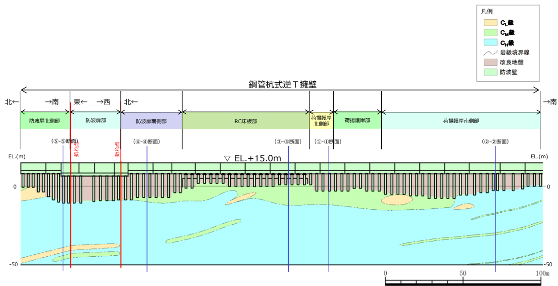
第6-11 図 防波壁（鋼管杭式逆T擁壁）の岩級縦断面図
