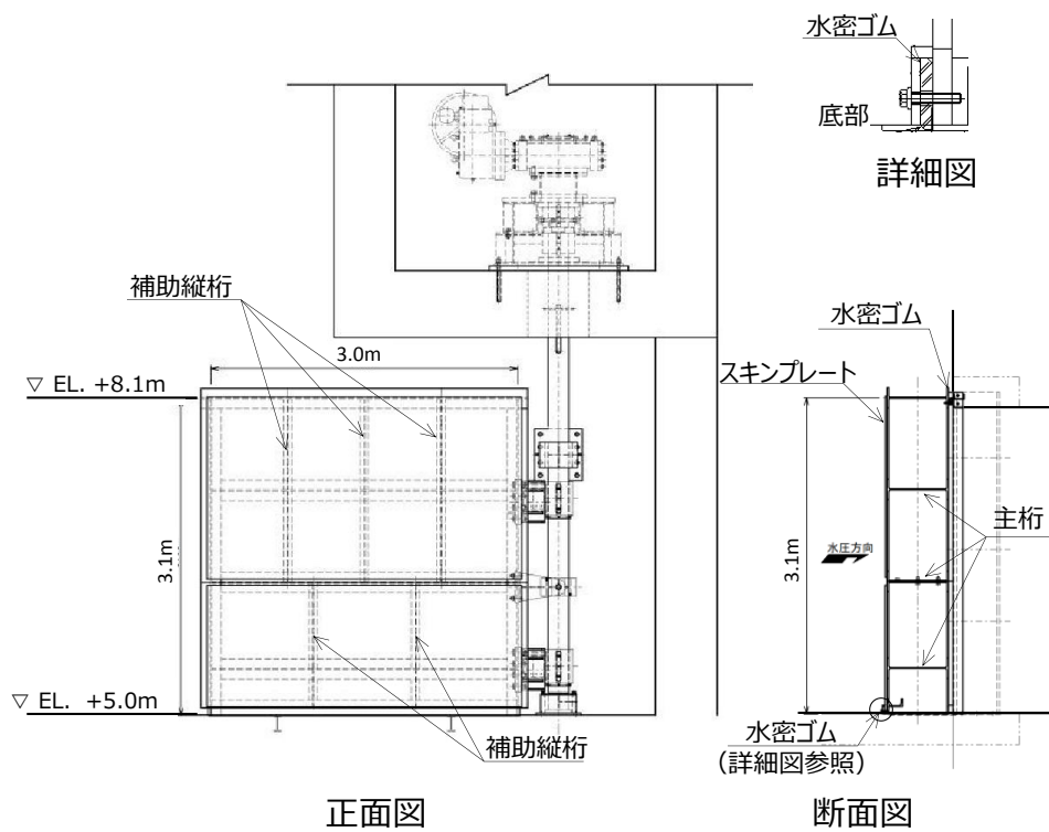
第 8-21 図 防波壁通路防波扉（1号放水連絡通路） 正面図・断面図
