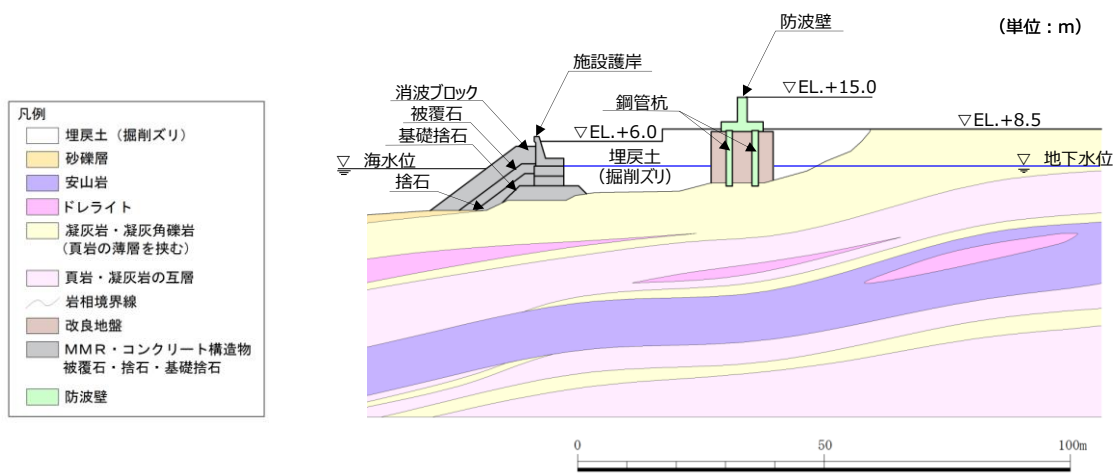
第6-12 図 防波壁（鋼管杭式逆T擁壁）の地質断面図（①-①）
