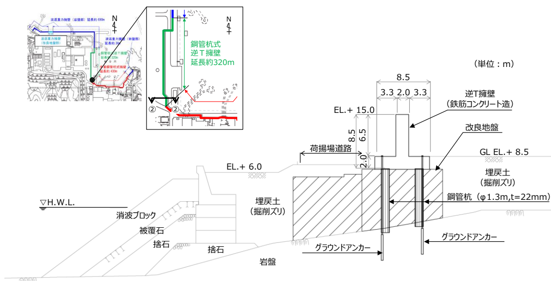
第 6-4(2) 図 防波壁（鋼管杭式逆 T 擁壁）荷揚護岸南側部 (②—②断面) 断面図
