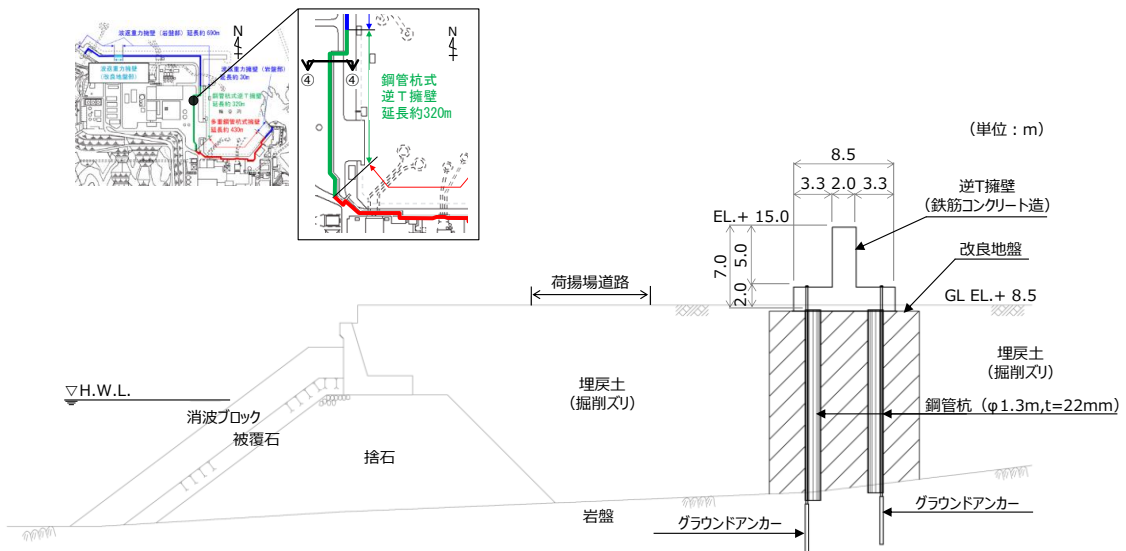
第 6-4(4) 図 防波壁 (鋼管杭式逆 T 擁壁) 防波扉南側部 (④-④断面) 断面図
