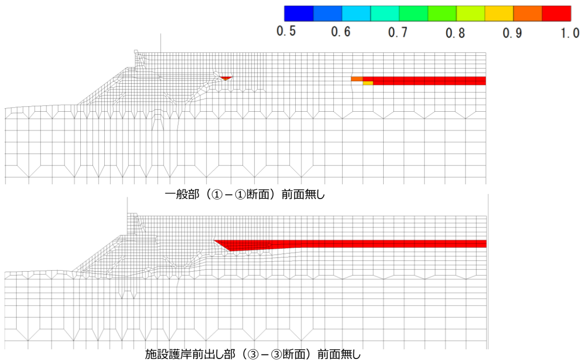
第 10-3-12 図 【参考】全時刻での過剰間隙水圧比の分布
