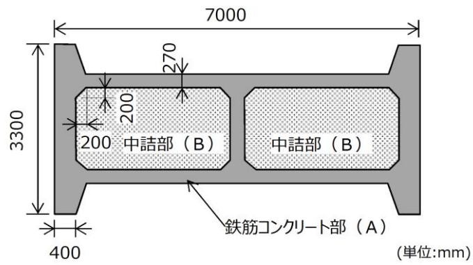
第9-26 図 セルラーブロック平面図 (例)
