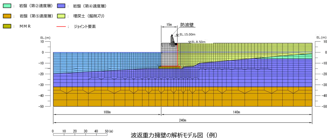
第7-23 図 防波壁（波返重力擁壁）の解析モデル
