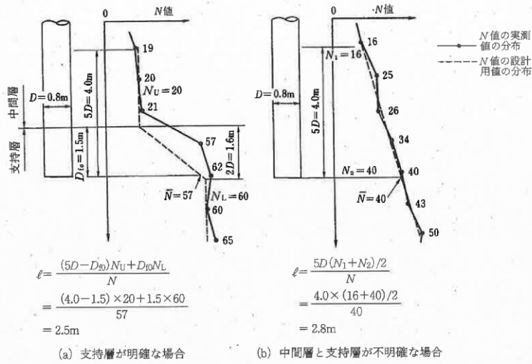
解説図 15.2.2.3-1 打込み杭工法による先端開放鋼管杭の支持層への換算根入れ深さ \ell
