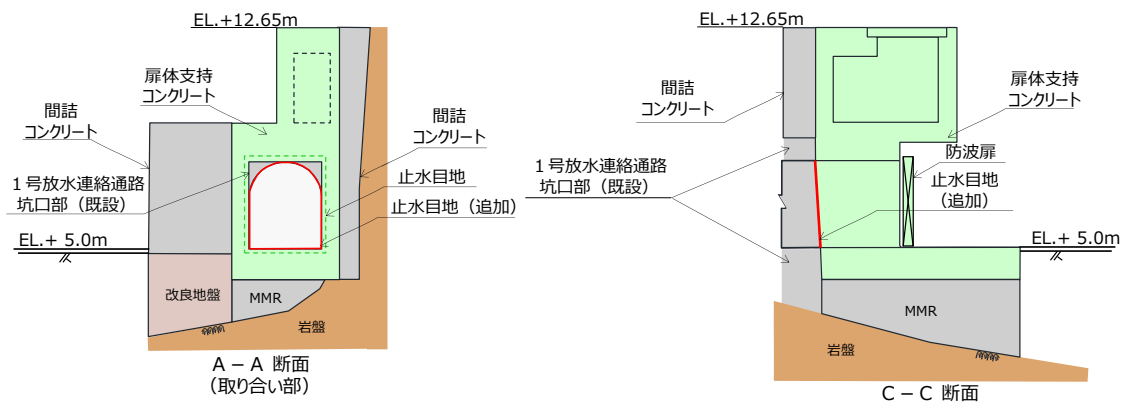
第 8-26 図 1 号放水連絡通路防波扉「施設」の範囲
