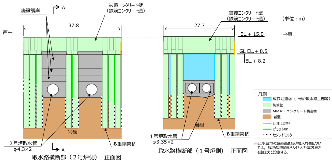
第 5-27 図 防波壁 (多重鋼管杭式擁壁) 弱部②概要図 (取水路横断面正面図)
