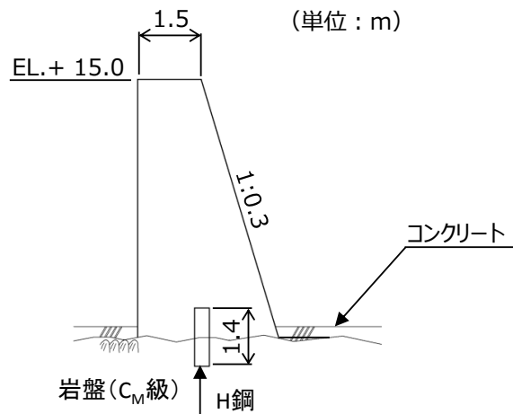
第 7-5(6) 図 防波壁 (波返重力擁壁) 西端部 (⑥-⑥) 断面図
