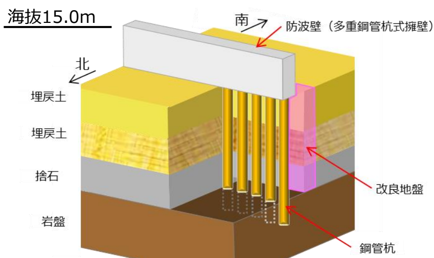
第4-2(1)図 防波壁（多重鋼管杭式擁壁）（岩盤支持）の評価対象部位
