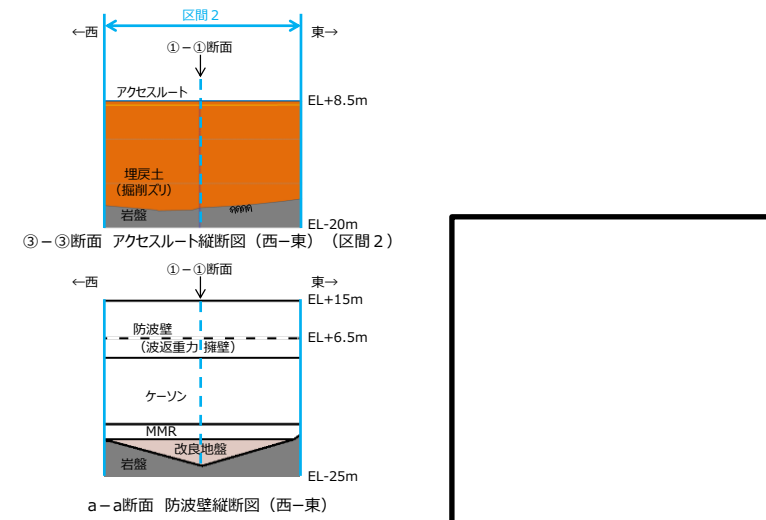
第4-24 図 防波壁（波返重力擁壁）（縦断面）
