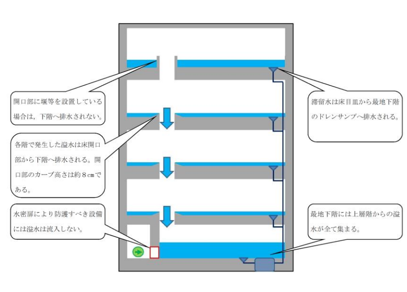
第2図 水位評価概要図
