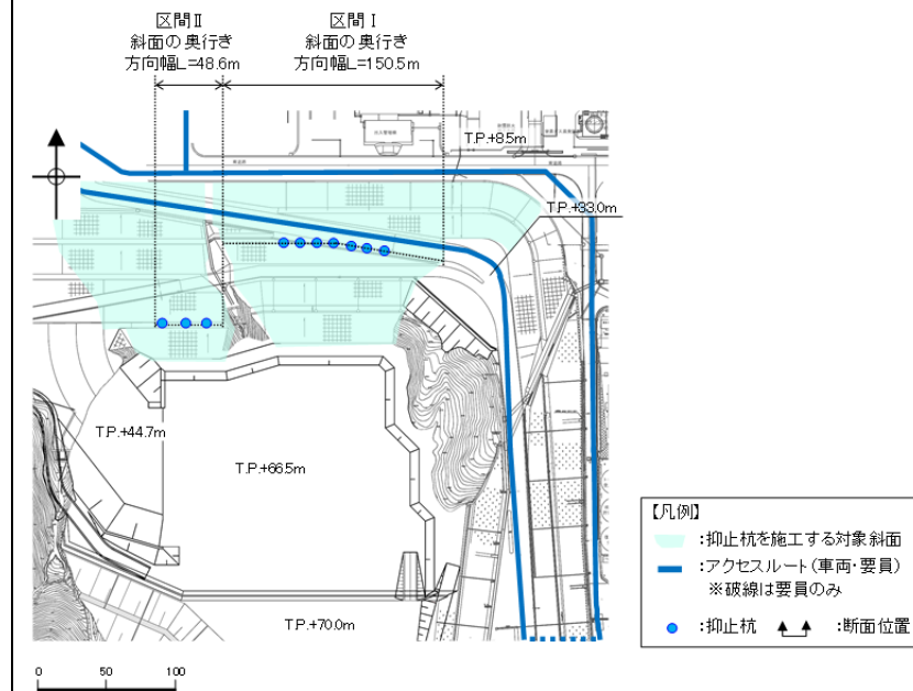
平面図
