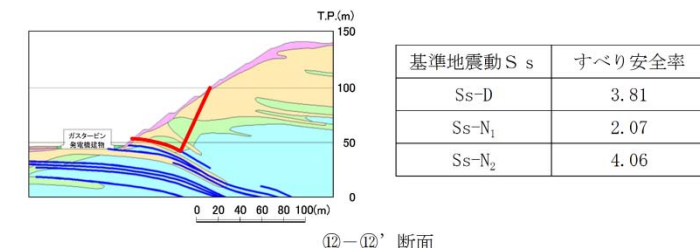
⑫-⑫' 断面
