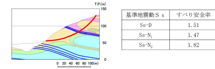
⑬-⑬' 断面
