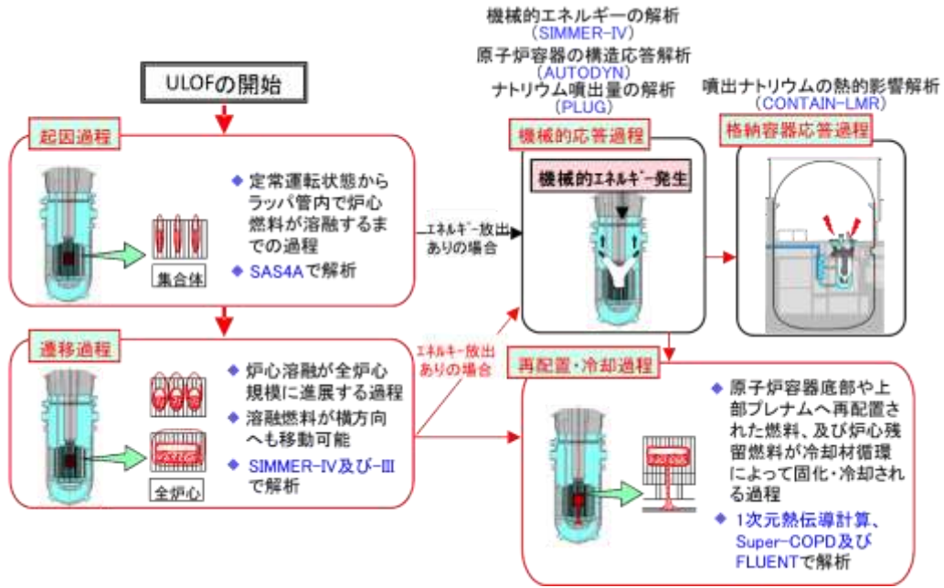
第 1. 1. 1 図 ULOF の事象進展と格納容器破損防止措置の有効性評価における解析の流れ
