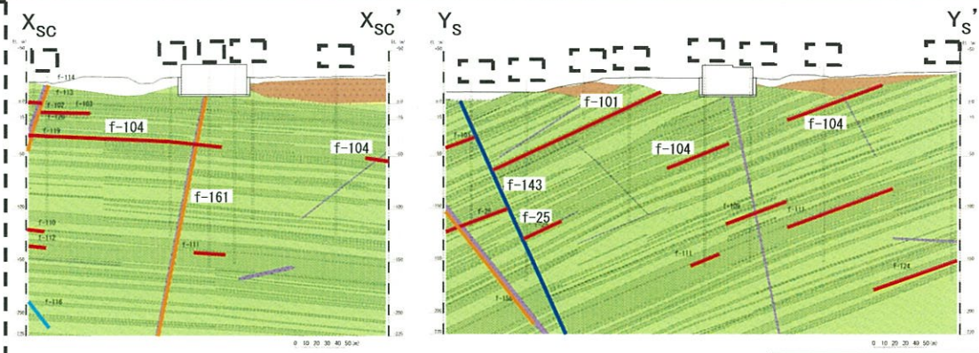
X_{SC}-X_{SC}' 断面 Y_S-Y_S' 断面 — タイプ①断層 — タイプ②-1断層 — タイプ②-2断層 — タイプ③断層
