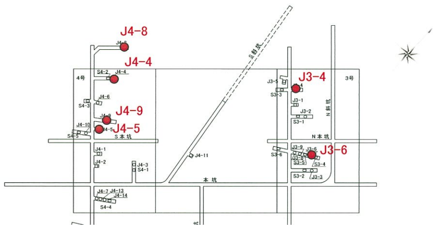
支持力試験位置図(3,4号試験坑平面図)
