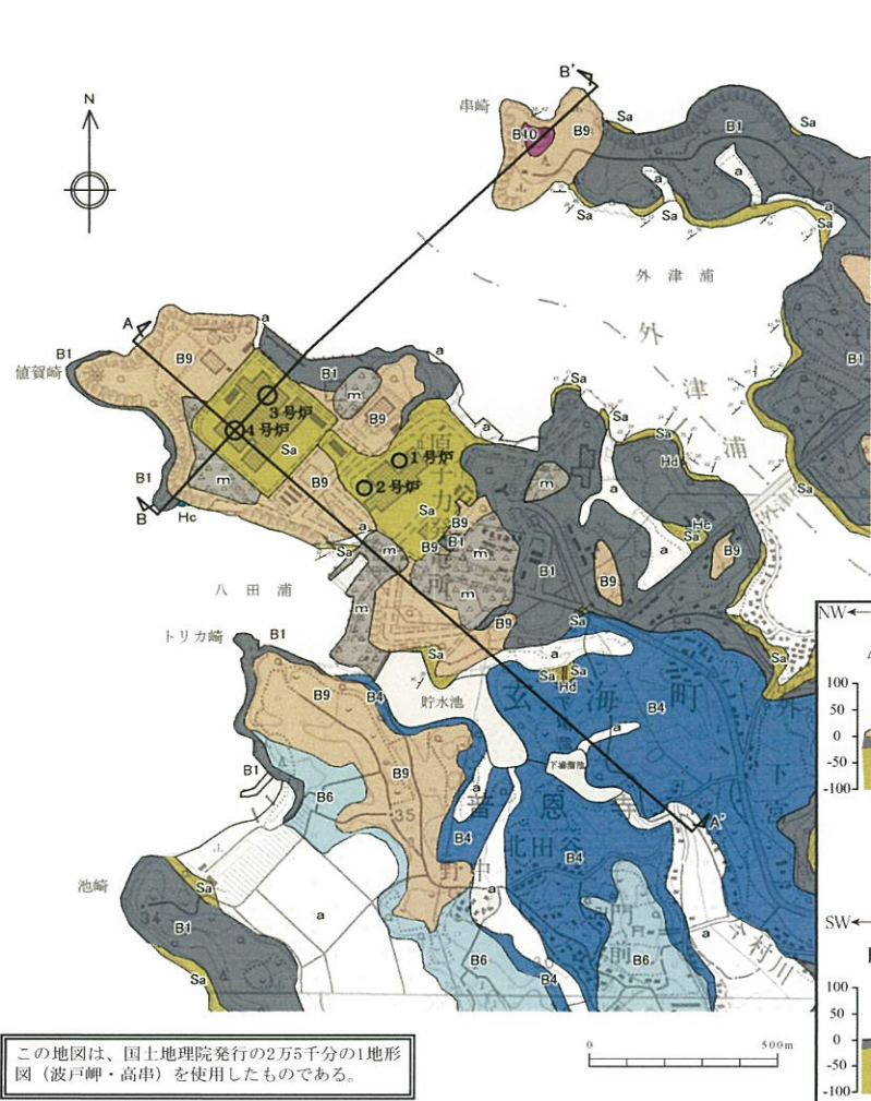
敷地内地質平面図
