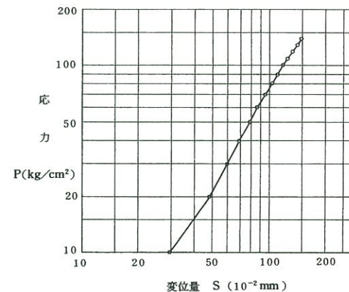
J3-6試験結果 (頁岩③級)
