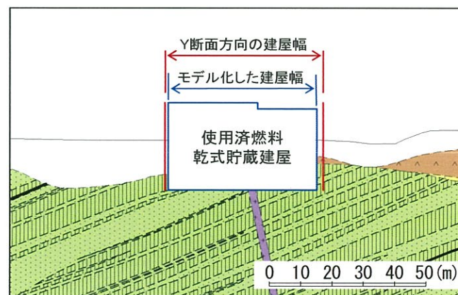
Y_S-Y'_S 断面(拡大図)
