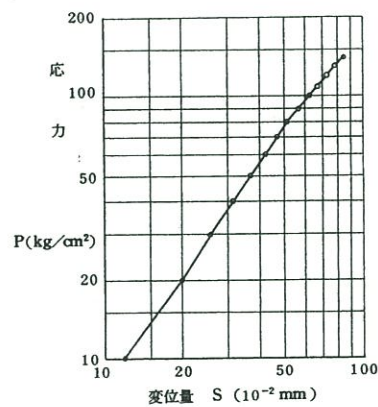
J4-8試験結果 (頁岩③級)
