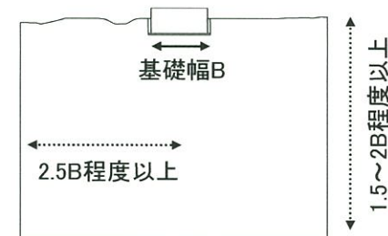
モデル領域設定の考え方
