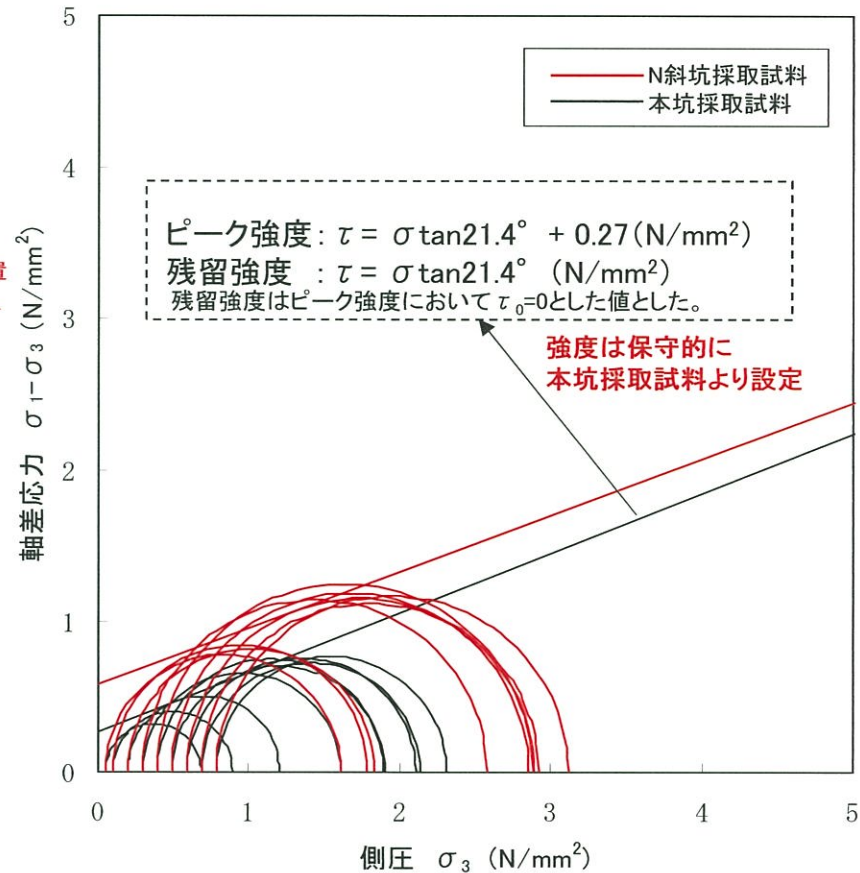
静的三軸圧縮試験結果
