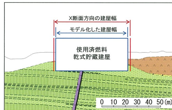
X_{SC}-X'_{SC} 断面(拡大図)
