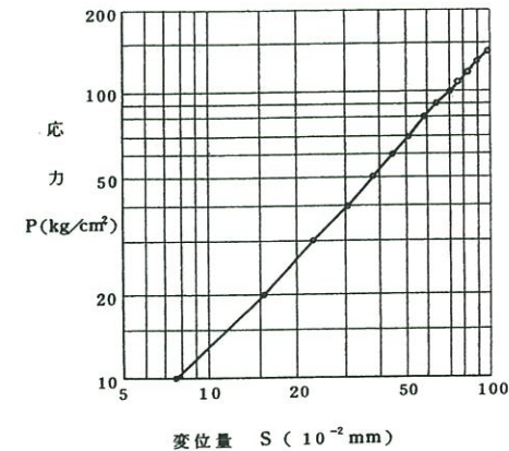
J4-9試験結果 (頁岩③級)
