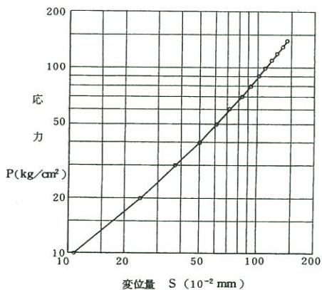
J4-4試験結果 (砂岩③級)
