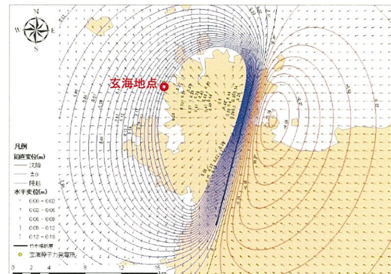
竹木場断層
