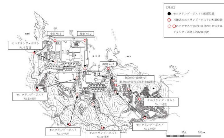
第5図 可搬式モニタリング・ポストの配置位置にアクセスできない場合の代替測定場所
