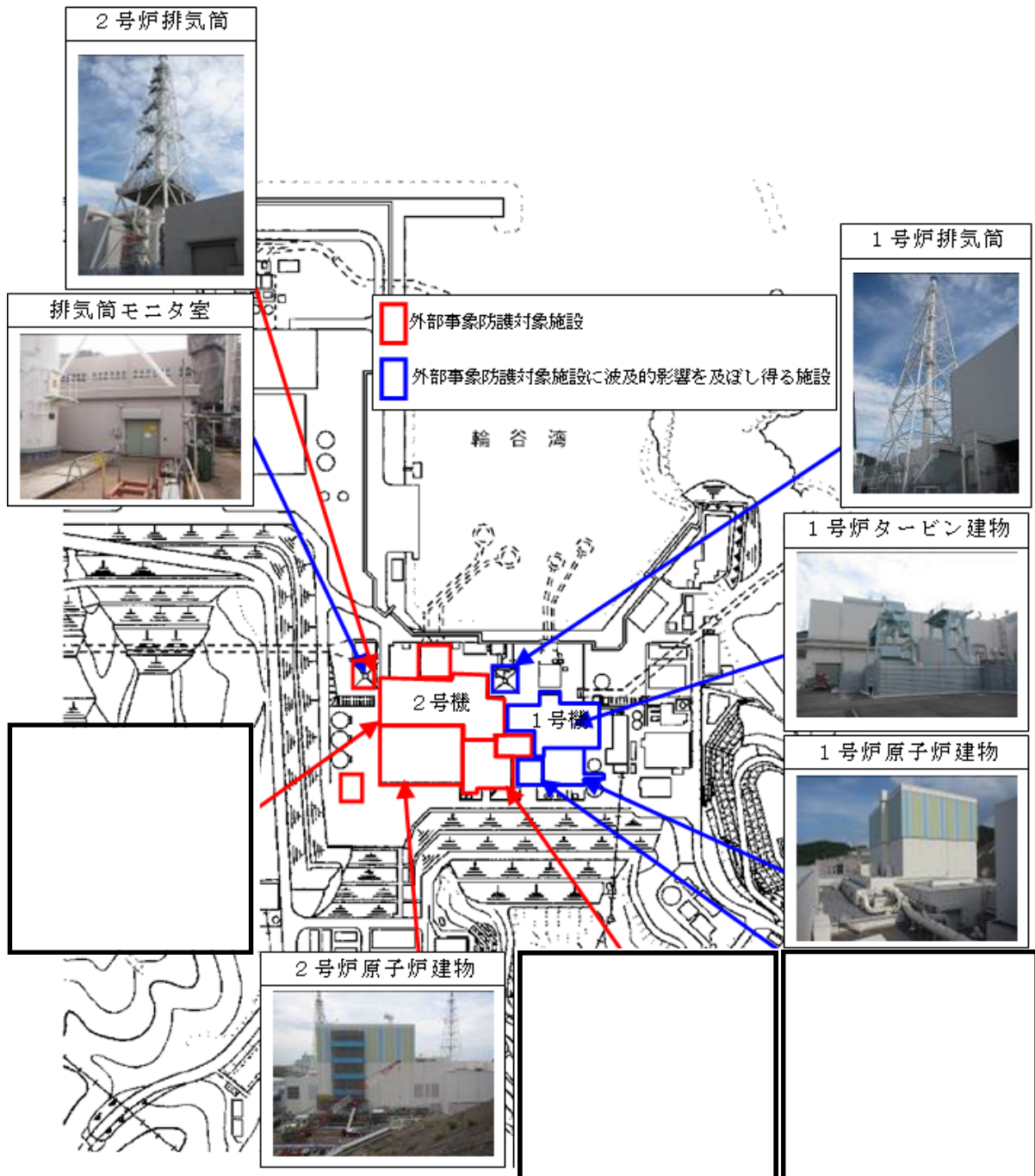
図 1.2.4 外部事象防護対象施設のうち評価対象施設及び外部事象防護対象施設に波及的影響を及ぼし得る評価対象施設の構内配置
