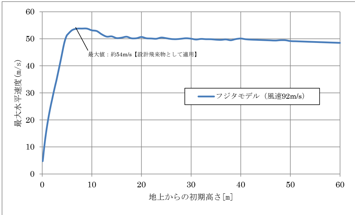
図2 砂利の飛散解析結果 (砂利：40mm×40mm×40mm, 0.2kg)
