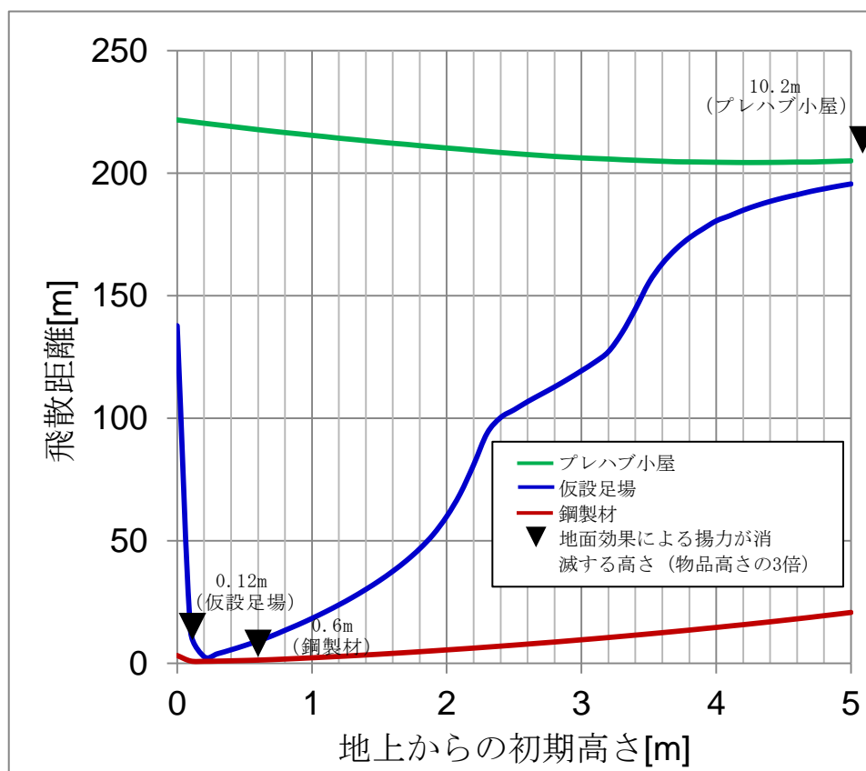
図1 プレハブ小屋（塊状），仮設足場（板状），鋼製材（棒状）の地上からの初期高さ と 飛散距離の関係
