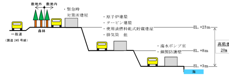
別図 3-1 評価対象施設及び防護対策設備と車両の存在場所との高さ関係
