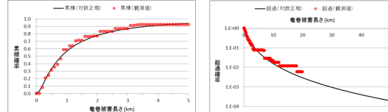
(a) 累積確率 (b) 超過確率 図 2.3.9 竜巻被害長さの確率分布の推定結果と観測値との比較
