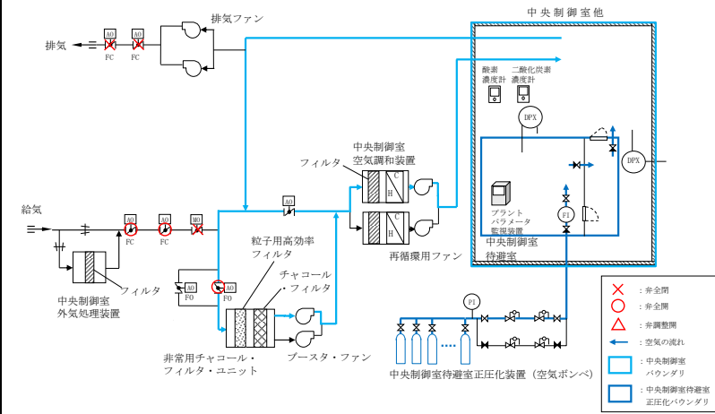
図3 (2 / 2) 中央制御室換気系及び中央制御室待避室正圧化装置 (空気ポンプ) 概略系統図 (非常時運転モード (加圧運転 (プルーム通過中)))
