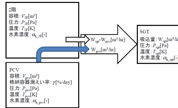
図 59-12-1 評価モデル
