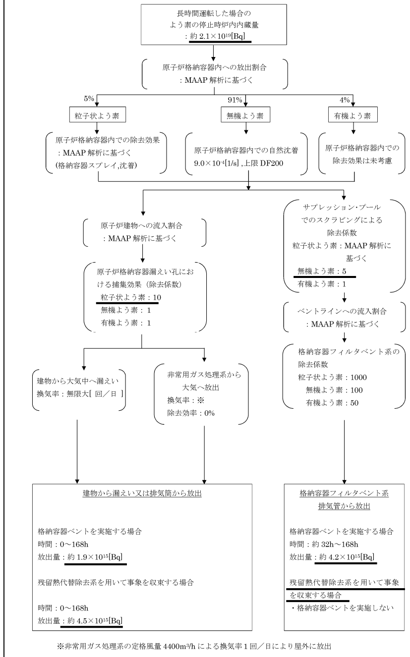
図 4-2 炉心の著しい損傷が発生した場合のよう素の大気放出過程
