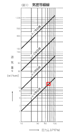
図 59-14-3 気密等級線図 (A4等級)
