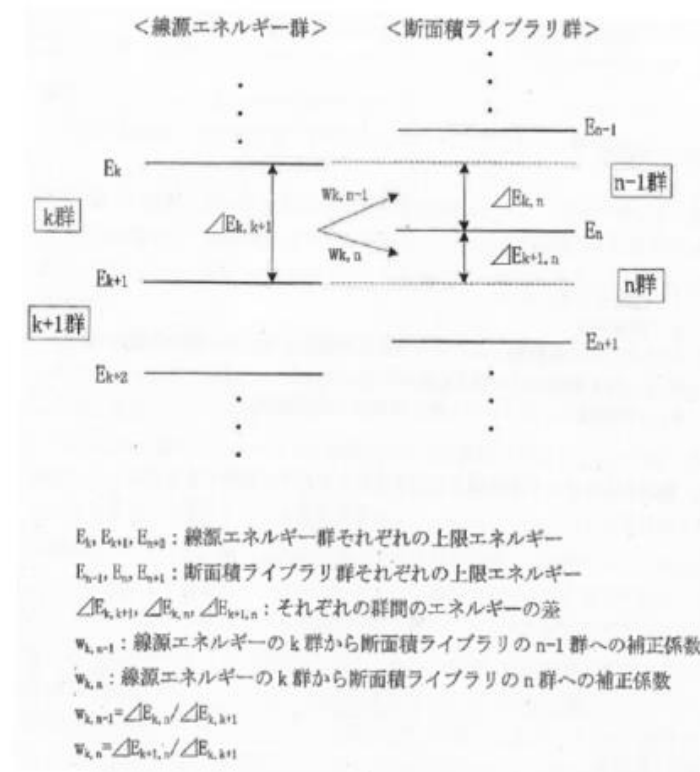
図 2-13-1 エネルギー群の変換方法
