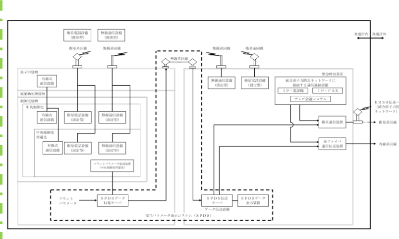
図 2.4-20 プラントパラメータ監視装置 (中央制御室待避室) のデータ伝送 概要図
